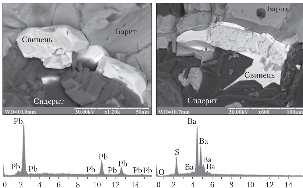
Рис. 2. Самородний свинець (білий) з баритом (світло-сірий) і сидеритом (темно-сірий) – полімінеральний цемент у порово-кавернозно-тріщинному просторі вторинного колектора (ДДЗ, св. 200-Східно-Павлівська, інт. 5280–5286 м)
