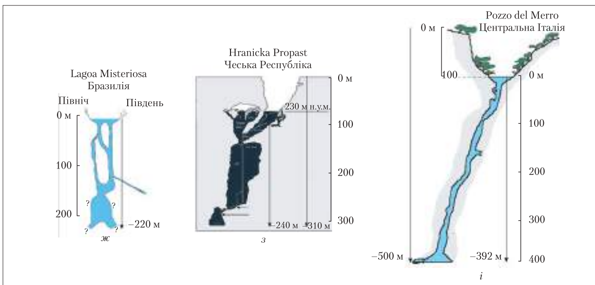
Рис. 6. Приклади щілиноподібних («рифтові») та округлих (шахти) субвертикальних каналів висхідних пере-токів (розвантаження) глибинних вод. Рифтові канали: а — активна (що розвантажує термальні води) печера Молнар Янош, Угорщина (фото А. Калинович); б — печера Девіс Хоул, Велика Британія (фото Е. Фарант); в–е — розкриті рифти: в, г — внутрішня гряда Передгірного Криму; д — район Жандайра на північному сході Бразилії; е — район Кейп у Південній Африці (рифт, що розкрився 07.01.2017 р. після інтенсивних опадів). Округлі канали: ж–і — найглибші в світі активні висхідні шахти в районі Бодогуена у Західній Бразилії ( ж ; [36]), Богемському масиві Чеської Республіки ( з ; [37]) і Апеннінах біля Риму в Італії ( і ; [38])
