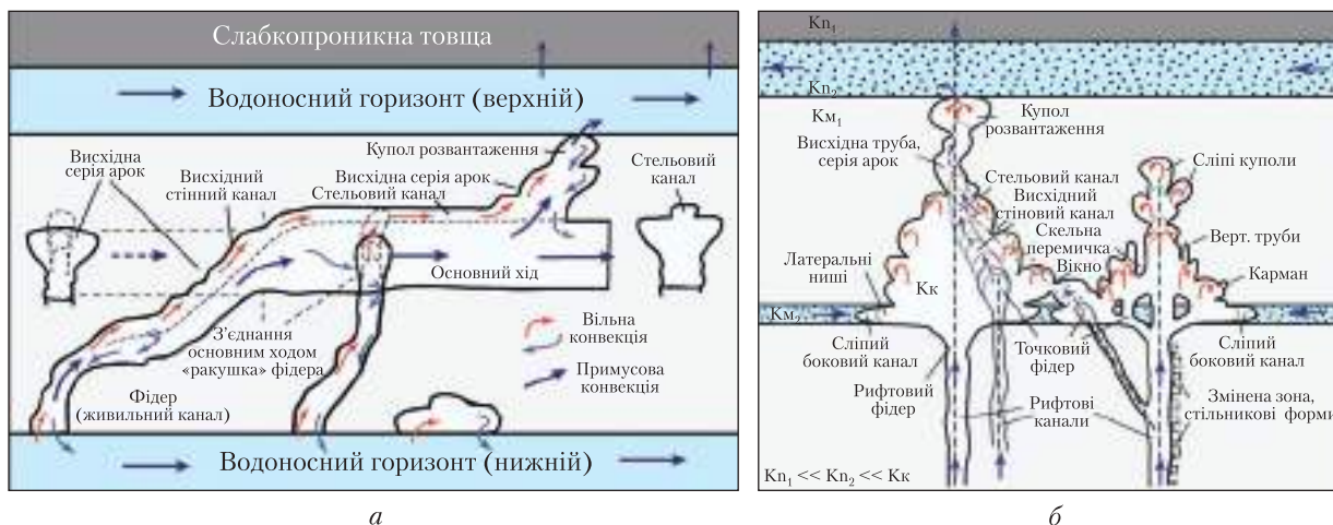
Рис. 9. Морфологічний комплекс висхідних потоків у каналово-порожнинних системах з домінуванням пластової (а) і кризьформаційної (б) організації. K_{n1} і K_{n2} — порова проникність різних шарів; K_k — проникність каналів
