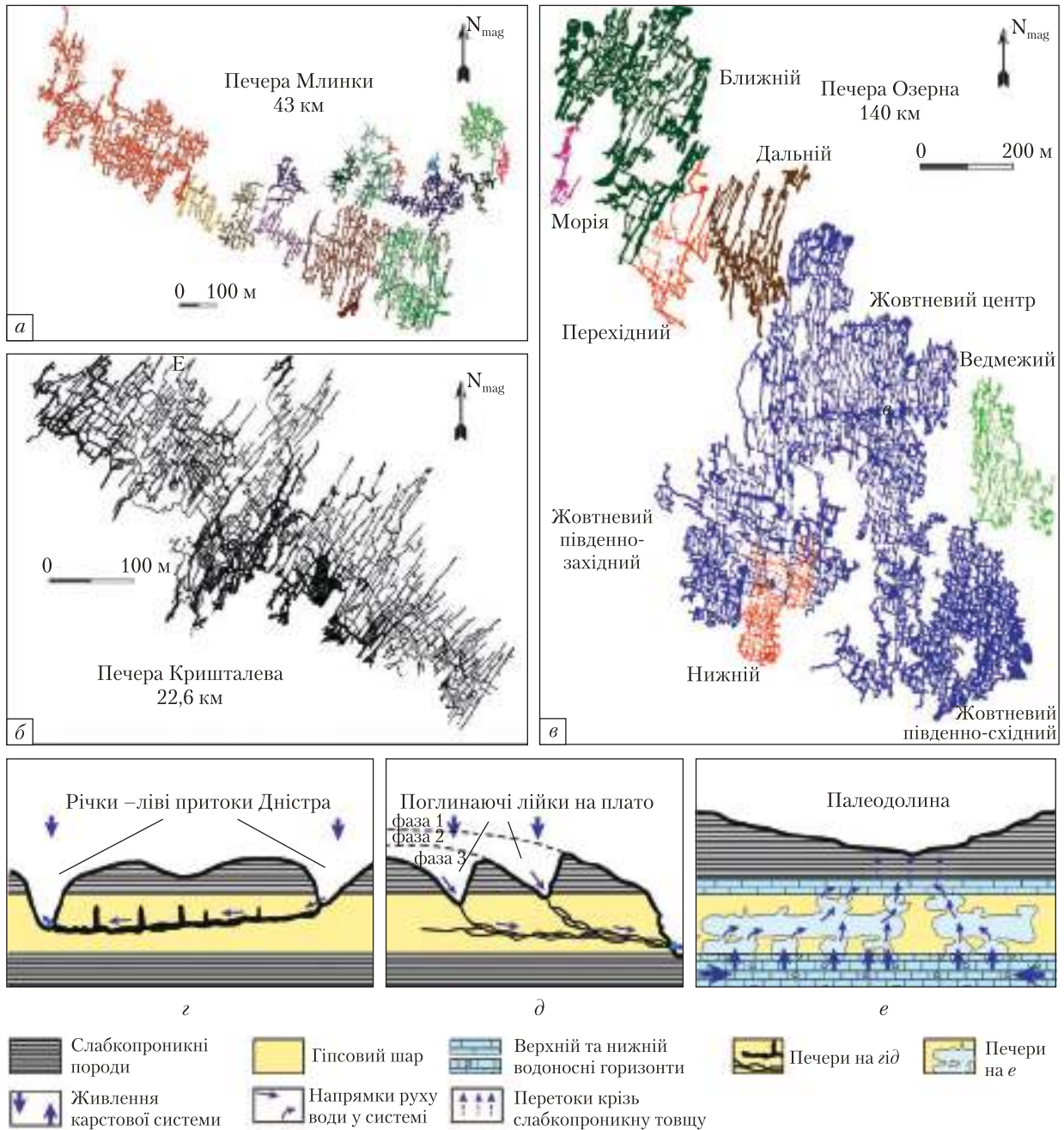
Рис. 5. Плани гігантських лабіринтових печерних систем у гіпсах Лівобережного Придністров'я та концептуальні моделі їх формування: а, б, в – плани печер за матеріалами спелеологічних клубів – чортківського «Кристал» і тернопільського «Поділля»; г – епігенна модель за [34]; д – епігенна модель за [35]; е – гіпогенна артезіанська модель за [15, 16]
