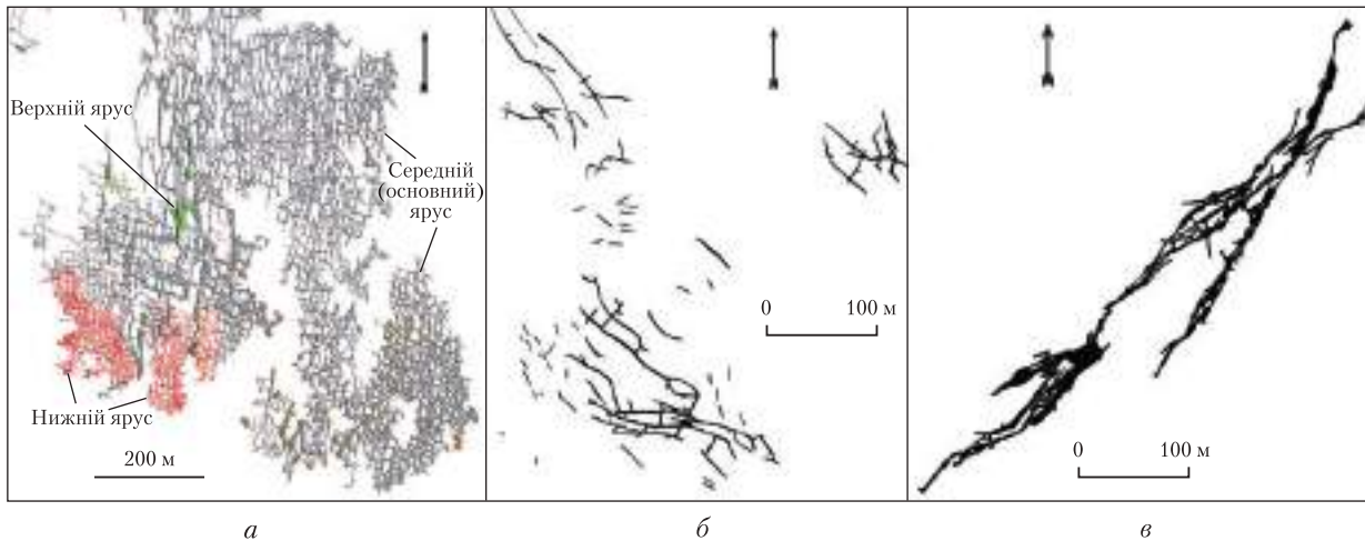
Рис. 4. Характерні структури гіпогенних каналово-порожнинних систем у плані: а, б — крізьпластового артезіанського спелеогенезу; в — крізьформаційного спелеогенезу з глибинним живленням. На ( а ) зображено фрагмент карти приблизно 50 км ходів печери Озерна, Західне Поділля, загальна довжина якої становить понад 130 км (зйомка Тернопільського спелеоклубу); на ( б ) — ізольовані канали та кластери каналів у понтичних вапняках Одеси [21]; на ( в ) — печера Сонора у південно-західному Техасі [22]
