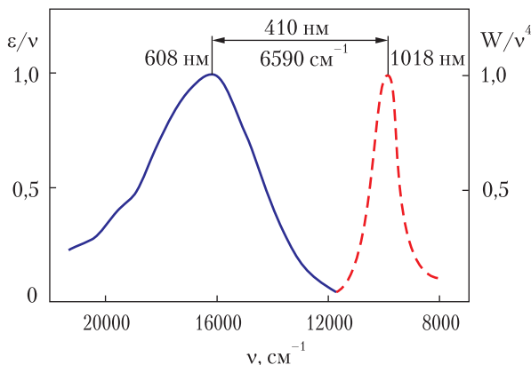
Рис. 2. Спектри поглинання і флуоресценції ПБ 15 в ацетонітрилі: \varepsilon — екстинкція, W — інтенсивність флуоресценції, \nu — хвильове число
