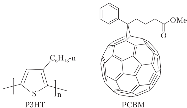
Рис. 8. Структурні формули полі-3- n -гексилтіофену (РЗНТ) і метилового естеру [6,6]-феніл- \text{C}_{61} -масляної кислоти (РСВМ)
