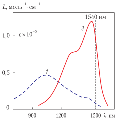
Рис. 4. Спектри поглинання ПБ 18 в ацетонітрилі (1) і о -дихлорбензолі (2)
