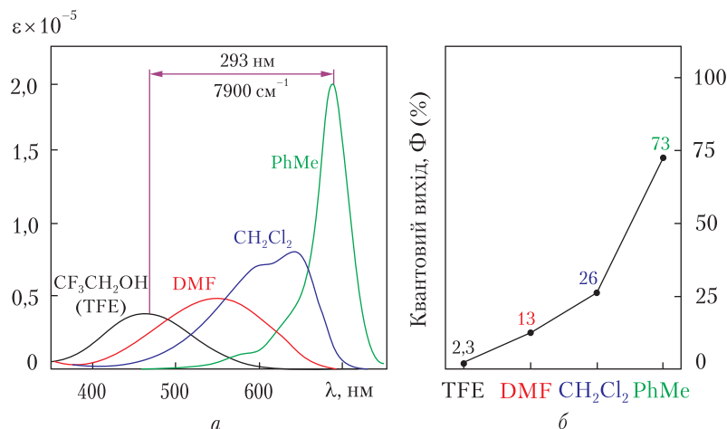
Рис. 3. Спектри поглинання (а) і квантові виходи флуоресценції (б) ПБ 17 у різних розчинниках
