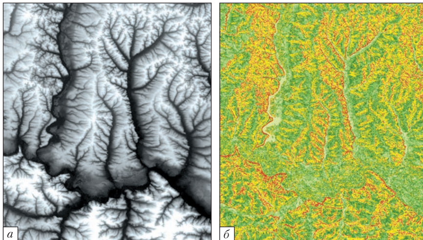
Рис. 2. Приклад використання методики для розрахунку індексу ER на території з координатами 37,22E 49,91N та 38,69E 48,64N у масштабі 1:500000: а — цифрова модель рельєфу DEM з просторовою роздільною здатністю 30 м; б — отримані за методикою значення індексу ER
