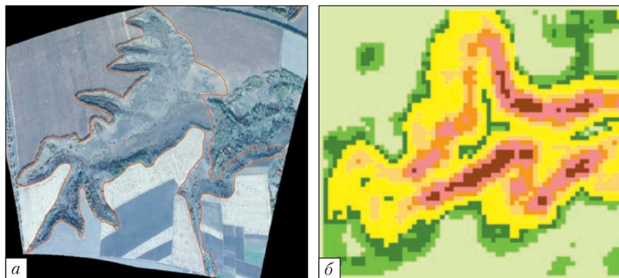
Рис. 4. Оцінка стану ерозійних процесів на землях сільськогосподарського призначення на модельному ярі Халчанської сільської ради Кагарлицького району Київської області: а — площа яру за супутниковим знімком з КА QuickBird від 14 жовтня 2014 р.; б — розрахунок індексу ER для цієї території за даними DEM
