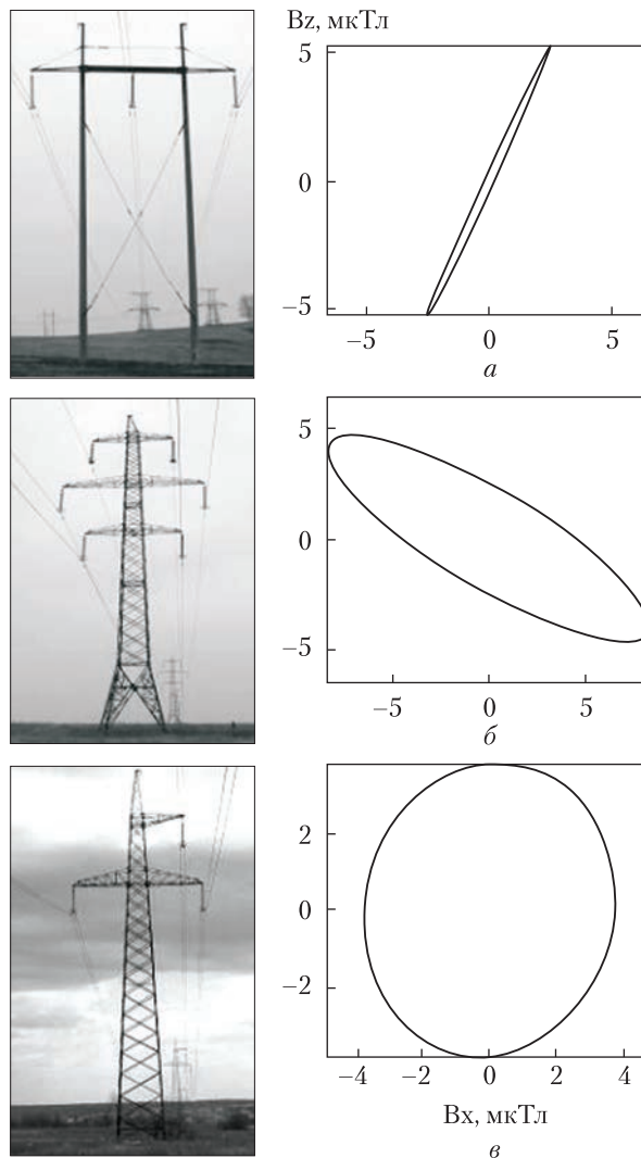
Рис. 3. Типи високовольтних ЛЕП, поширені в Україні: a — горизонтальний підвіс проводів; b — вертикальний підвіс проводів; v — підвіс проводів типу «трикутник» та відповідні годографи вектора магнітного поля
