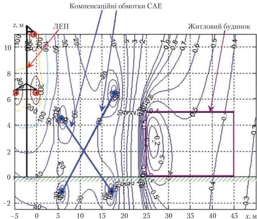
Рис. 4. Розподіл індукції магнітного поля (мкТл) при використанні синтезованої системи активного екранування
