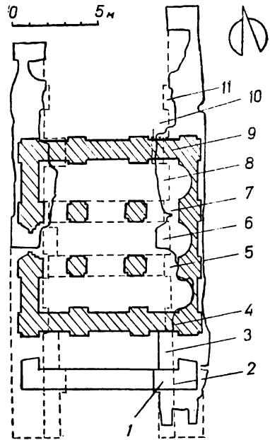
Рис. 1. Обмірний план Золотих воріт з сумішним планом надбрамної церкви. Реконструкція автора.
