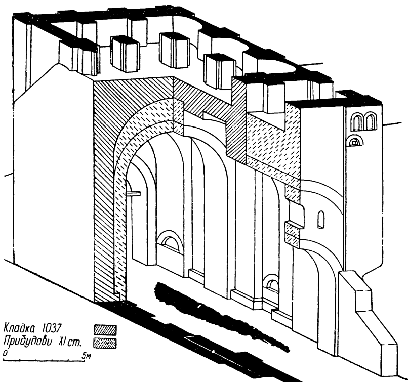
Рис. 3. Аксонометричний малюнок нижньої частини Золотих воріт. Спроба реконструкції автора.
