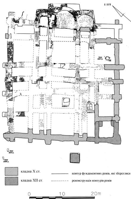
Ілюстр.4 План залишків Десятинної церкви Х–ХІІІ ст., складений за результатами розкопок 2005–2011 рр.
