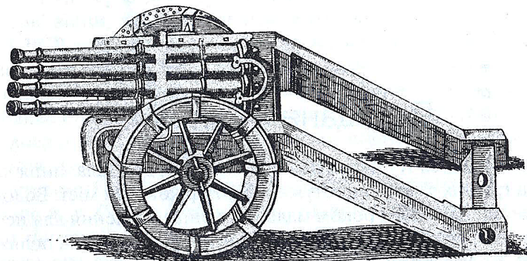
Багатоствольна гармата (ожига). Малюнок з артилерійського трактату. XVII ст. (фото: Ліпа К. Під захистом мурів (З історії української фортифікації X–XVII ст.). – К., 2008. – С.163)
