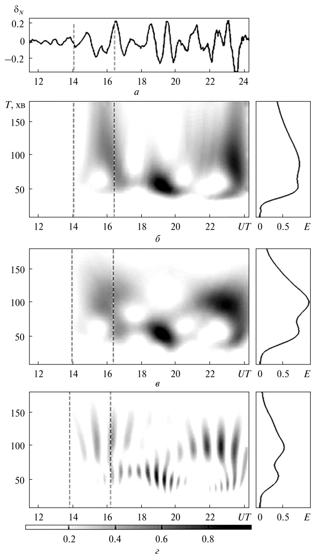
Рис. 30. Результати спектрального аналізу часових варіацій \delta_N(t) 8 листопада 2004 р. для висоти 200 км: a — сигнал, b , v , z — спектрограми сигналу (у відносних одиницях) відповідно віконного перетворення Фур'є, адаптивного перетворення Фур'є і вейвлет-перетворення, справа — енергограми сигналу у відносних одиницях
