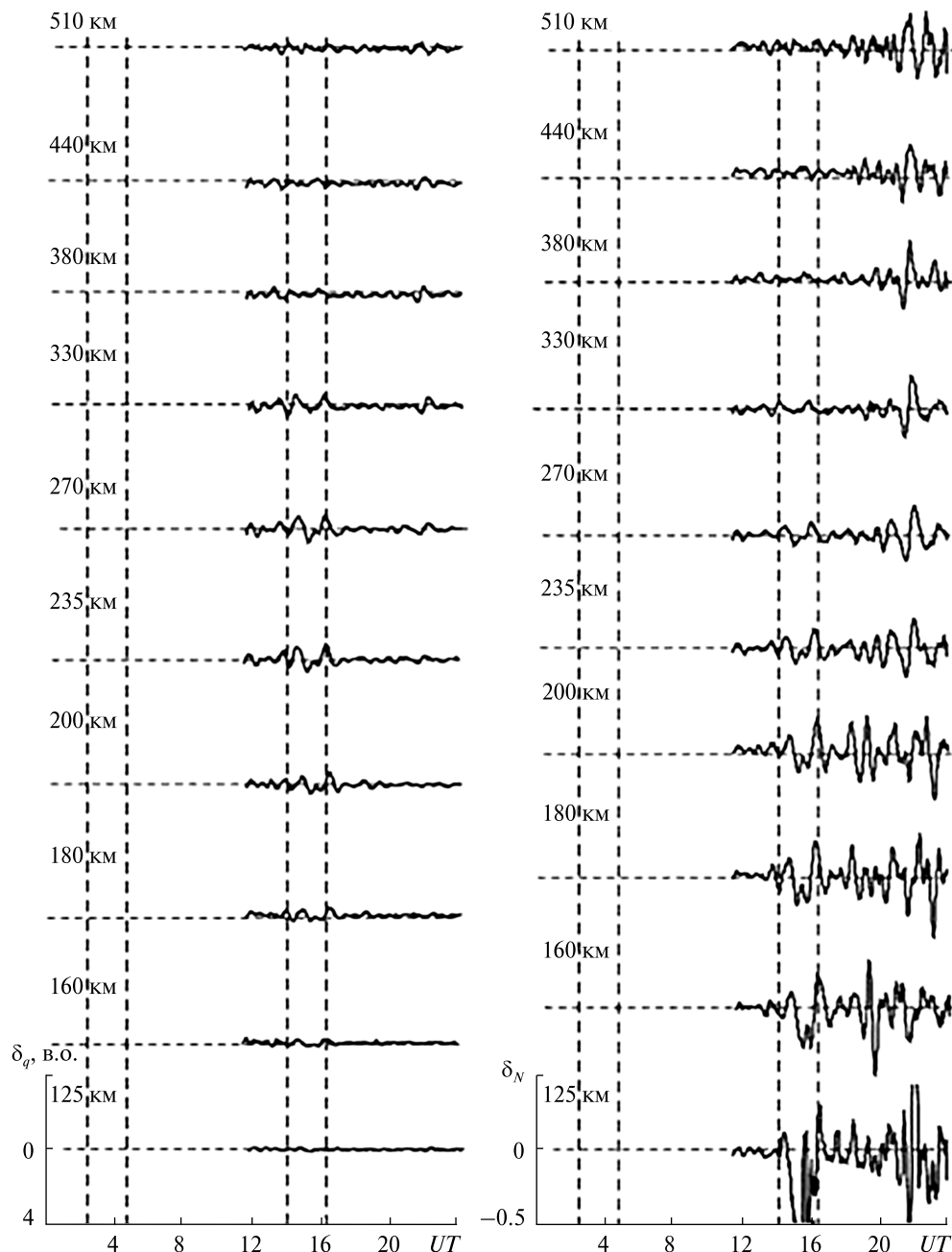
Рис. 25. Часові варіації збурень \delta_q і відносних збурень \delta_N концентрації електронів під час ІБ 8 листопада 2004 р. (вертикальні штрихові лінії — моменти сходу і заходу Сонця на висоті 450 км і на поверхні Землі)
