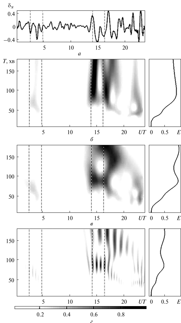
Рис. 31. Те ж, що на рис. 30, для 9 листопада 2004 р.
