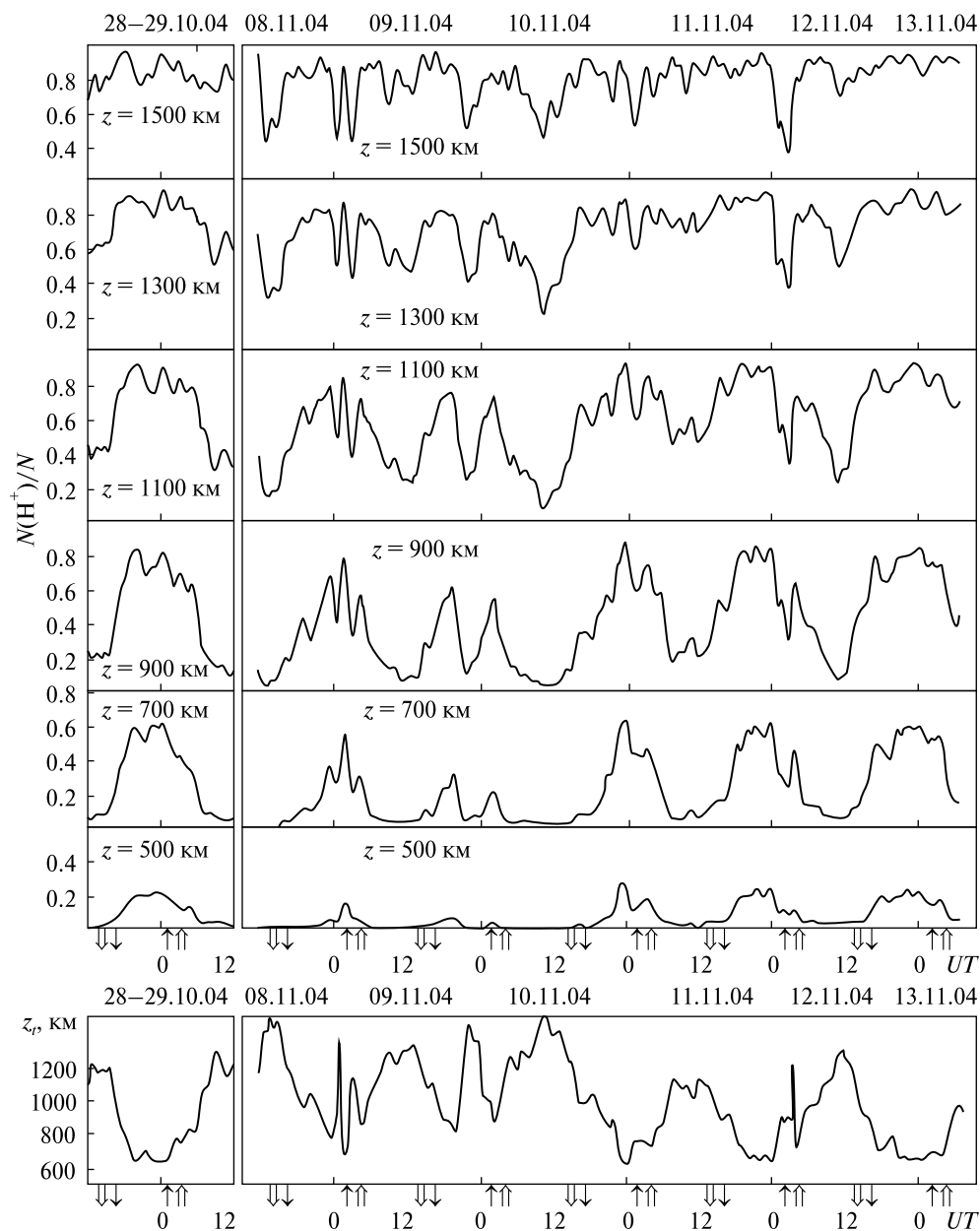
Рис. 24. Часові варіації відносної концентрації іонів водню N(\text{H}^+)/N на фіксованих висотах, де N(\text{O}^+) = N(\text{H}^+) , і висоти z_i (нижня панель) в контрольну добу 28-29 жовтня і в збурений період 8...13 листопада 2004 р. (зовні усереднення на інтервалі 105 хв з кроком 15 хв)
