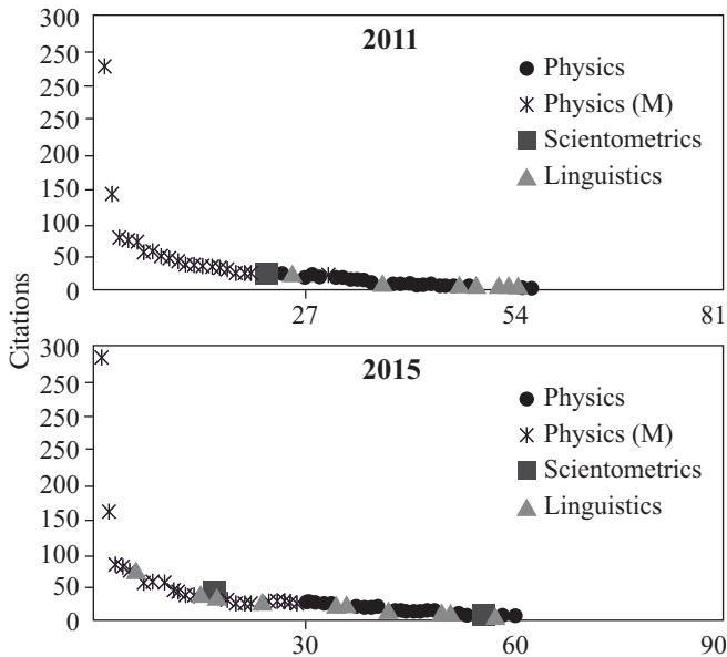
Рис. 4. Тематичне ядро публікацій Попеску за 2011 та 2015 роки. З-поміж публікацій з фізики (Physics) виокремлено основні (main) тематичні публікації тематичного ядра 2018 року, Physics (M)
