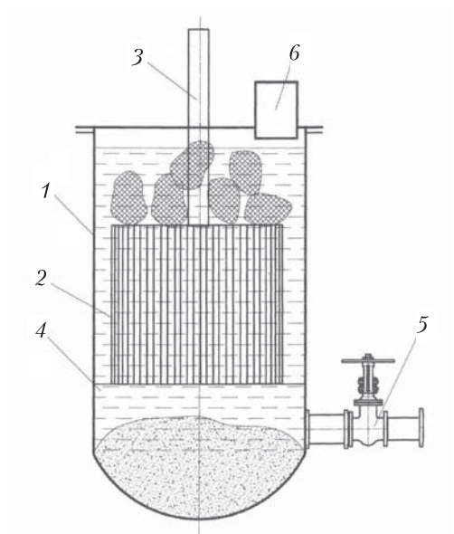
Рис. 3. Конструктивная схема технологического узла: 1 – корпус разрядной камеры; 2 – щелевой классификатор; 3 – электродная система; 4 – сборник; 5 – система водоснабжения; 6 – загрузочное отверстие
