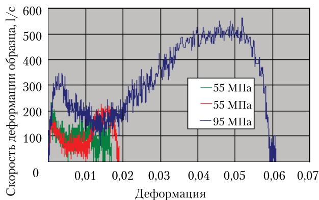
Рис. 2. Диаграмма скорости деформации металлургического кремния
