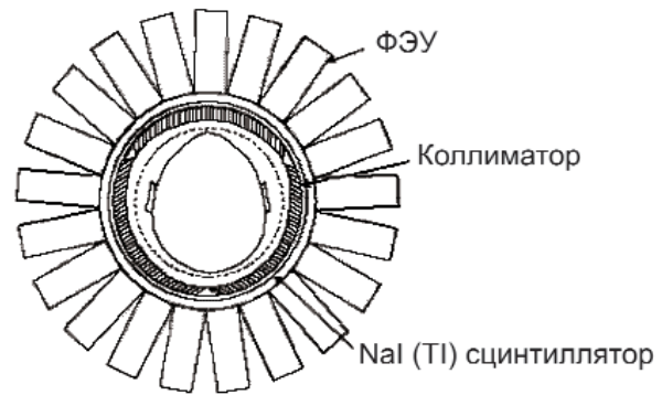
Рис. 1. Схема детектирования излучения в гамма камере "ОФЭКТ-3"
