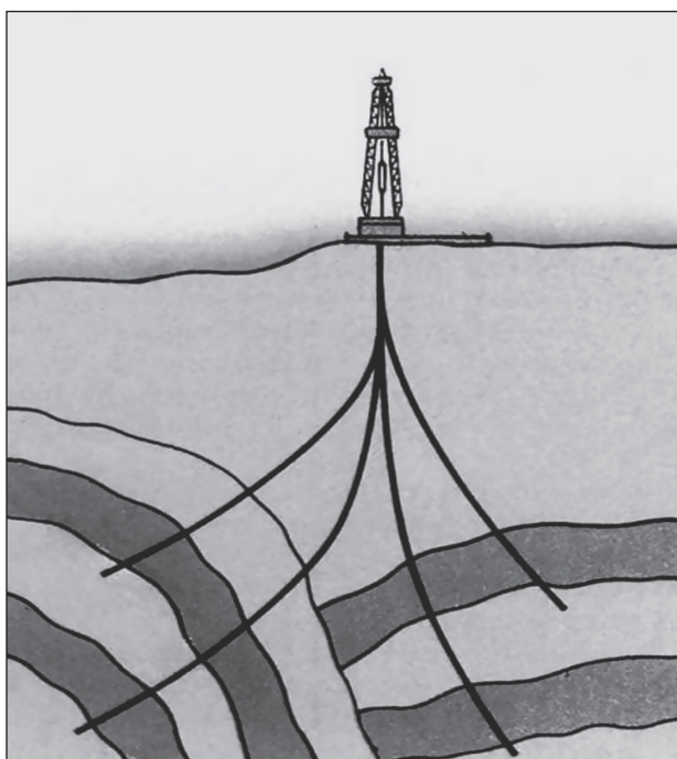
Рис. 5. Схема МБС
