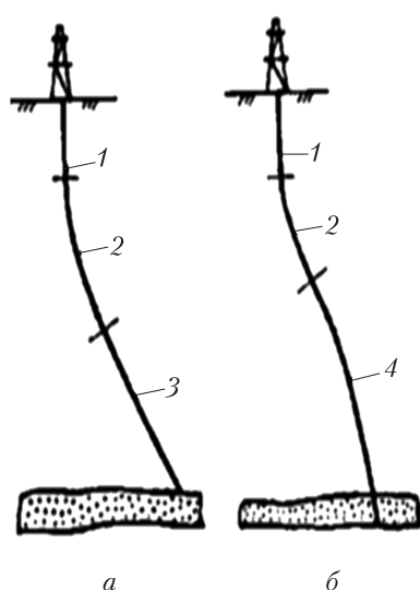
Рис. 3. Схема ННБ
