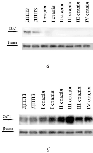
Рис. 2. Вестерн-блот-аналіз вмісту СПС (а) та САТ1 (б) доброякісних і злоякісних пухлинах
