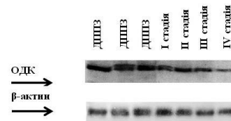
Рис. 1. Вестерн-блот-аналіз вмісту ОДК в доброякісних та злоякісних пухлинах ПЗ
