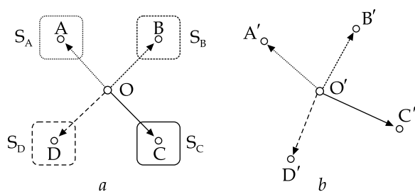
Рис. 1. Схема процесу формування векторів зіставлених віртуальних точок еталонного (а) і поточного (b) зображень
