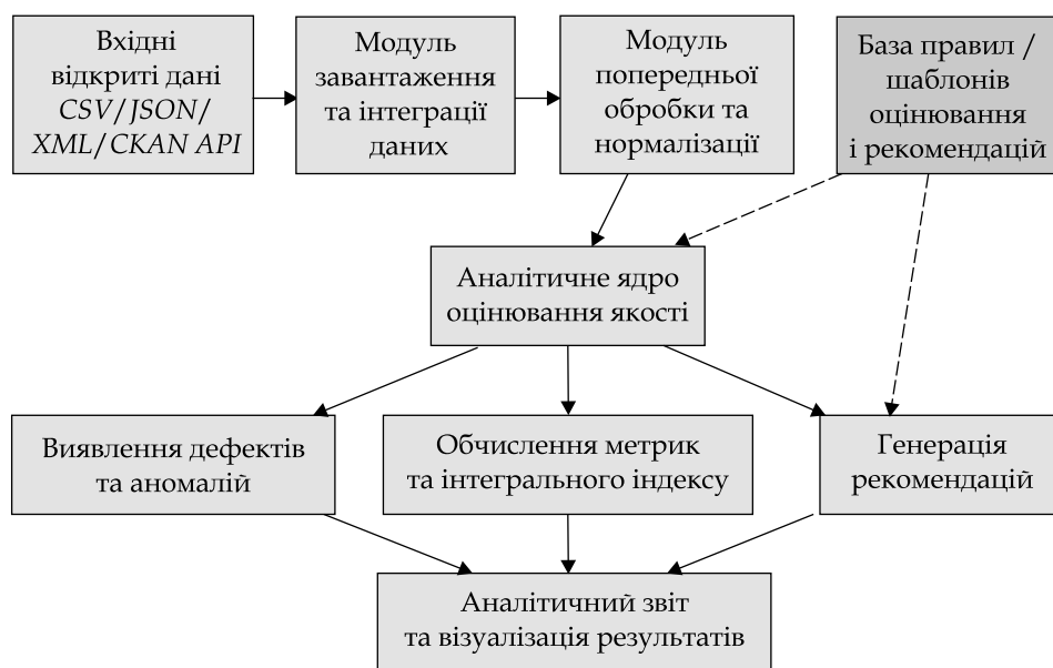
Рис. 1. Архітектура програмної системи інтелектуального оцінювання якості відкритих даних
