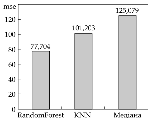
Рис. 4. Порівняння ефективності методів відновлення пропущених значень за метрикою RMSE
