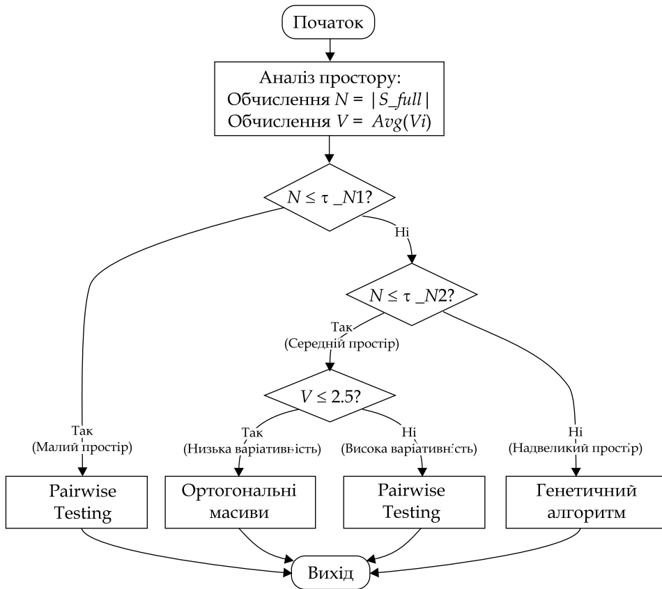
Рис. 1. Блок-схема адаптивного вибору методів оптимізації підсистемою маршрутизації (на рис. 1 англ. літери прокурсивити)
