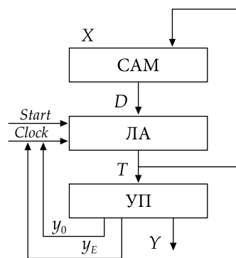
Рис. 1. Структурна схема КМПУ U_1
