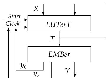
Рис. 3. Структурна схема F -КМПУ U_1
