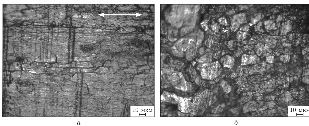
Рис. 4. Характерные виды деформационного рельефа, образовавшегося на поверхности рабочей части образцов сплава 1933, продеформированных до разрушения в оптимальных условиях ВССП. Направление растяжения образцов горизонтальное. Световая микроскопия
