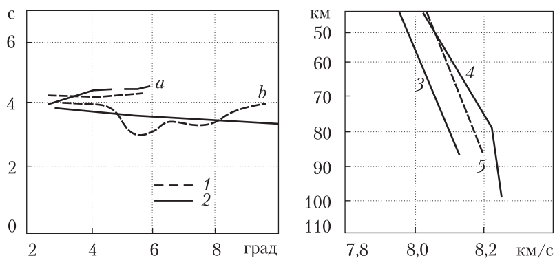
Рис. 3. Годографы для зон СА (а) и остальной части Украины, включающей платформенные и активизированные районы (б), и скоростные разрезы верхов мантии. Годографы: 1 — экспериментальные, 2 — расчетные. Скоростные разрезы: 3 — зон СА, 4 — “смеси” платформенных и активизированных зон, 5 — средний разрез для платформы и зоны СА Украины с использованием данных рис. 2, а
