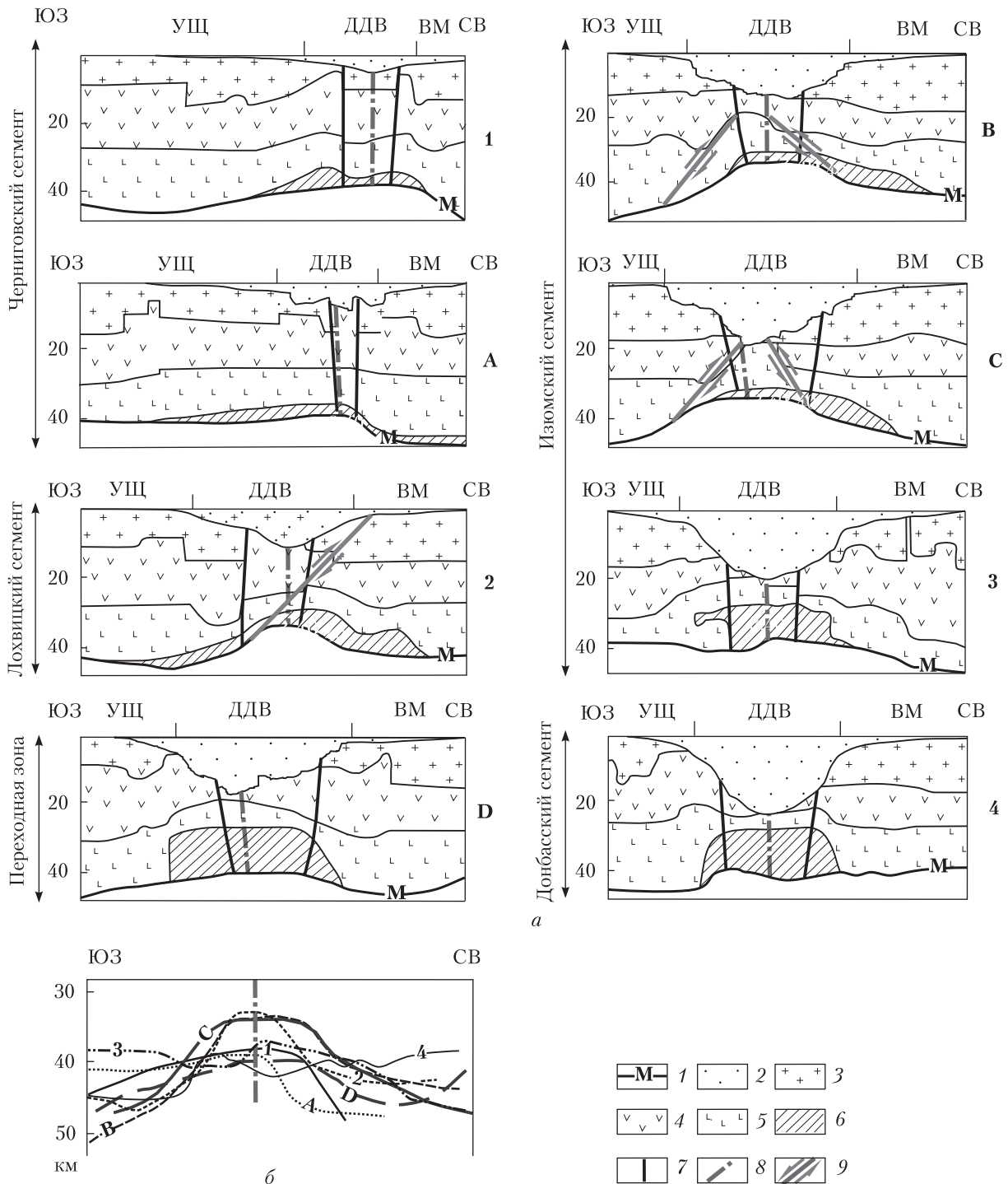
Рис. 4. Генерализованные разрезы земной коры вкост ДДВ (а) и поведение раздела Мохо относительно оси рифта по разрезам (см. номера на кривых) (б). 1 – положение раздела Мохо; 2 – осадочный, 3 – “гранитный”, 4 – “диоритовый”, 5 – “базальтовый”, 6 – коромантийная смесь; 7 – краевые разломы осевой части рифта; 8 – ось рифта; 9 – предполагаемые разломы внутри литосферы с направлением перемещений
