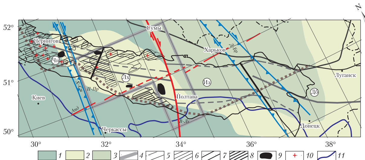
Рис. 3. Схема скоростной неоднородности подкоровой мантийной части литосферы ДДВ на глубинах 50 – 250 км и областей девонского магматизма по [7]. 1 – области повышенных значений аномалий скорости; 2 – области пониженных значений аномалий скорости; 3 – область переслаивания слоев положительных и отрицательных аномалий скорости; 4 – область сверхглубинных мантийных флюидов; 5 – щелочно-ультрамафическая пирокластика, переслаивающаяся с осадками; 6 – щелочно-ультраосновные лавы и пирокластика; 7 – мафические лавы, пирокластика, переслаивающаяся с осадками; 8 – мафические лавы и пирокластика; 9 – штоки; 10 – вулканические центры; 11 – граница распространения коромантийной смеси по изолинии \rho = 3,04 \text{ г/см}^3 . Другие условные обозначения см. на рис. 1, 2
