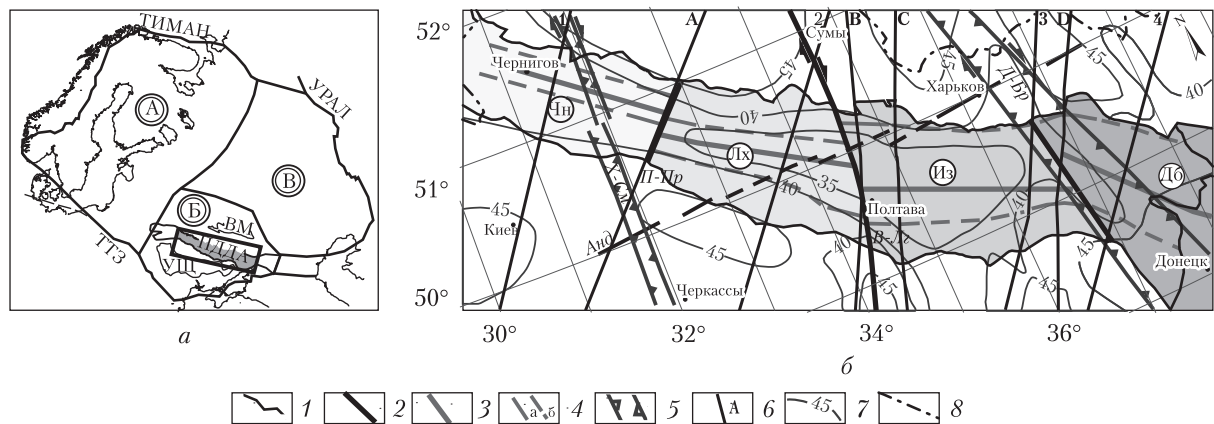
Рис. 1. Положение ДДВ в структуре Восточно-Европейского кратона (а) и ее сегментация по [4] (б). 1 – граница ДДВ; 2 – границы главных сегментов впадины; 3 – ось девонского рифта; 4 – границы центрального рифта: по данным [2] (а), по комплексу геофизических данных (б); 5 – трансрегиональные тектонические швы: Х-См – Херсон–Смоленск, Д-Бр – Донецк–Брянск; 6 – разрезы литосферы: по данным [2] (А, В, С, D), расчетные (1–4); 7 – изолинии глубины залегания раздела Мохо (км); 8 – государственные границы. Главные сегменты в пределах ДДВ (буквы в кружках): Чн – Черниговский, Лх – Лохвицкий, Из – Изюмский, Дб – Донбасс. Сегменты Восточно-Европейского кратона (буквы в двойных кружках): А – Фенноскандия, Б – Сарматия, В – Волго-Уралья. Разломь: П-Пр – Переяслав-Хмельницкий–Прилуцкий, В-Лг – Верховцевско-Львовский, Анд – Андрушевский. Сокращения: УЩ – Украинский щит; ВМ – Воронежский массив; ПДДА – Припятско-Днепровско-Донецкий авлакоген; ТТЗ – зона Тейсейра–Торнквиста. Площадь исследования в прямоугольнике (а)
