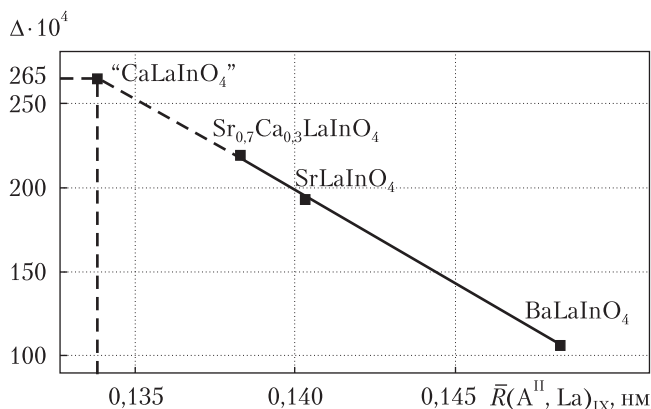
Рис. 2. Залежність ступеня деформації ( \Delta ) полієдрів (A^{II}, La)O_9 в ШПС A^{II}LaInO_4 від середнього кристалічного іонного радіуса атомів А-позиції ШПС R(\bar{A}^{II}, Ln)_{IX} . У роботі використана система кристалічних іонних радіусів [10]
