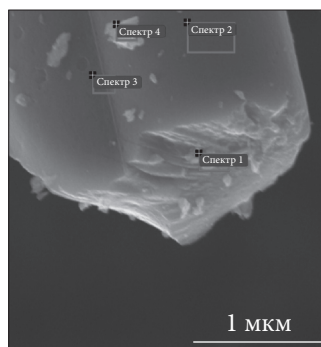
Рис. 2. Морфологія поверхні та елементний склад включень (мас. %) у довільно обраних точках для зразків КХАК V_s = 0,3 \text{ см}^3/\text{г} + 1 \% COS після інкубування в дистильованій воді протягом 24 год
