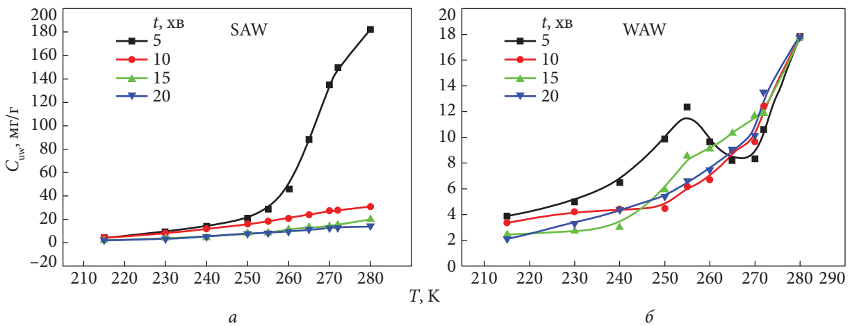
Рис. 3. Зміна концентрації сильно- та слабоасоційованої води залежно від температури і тривалості механічного оброблення ( t ) гідратованого метилкремнезему АМ-1
