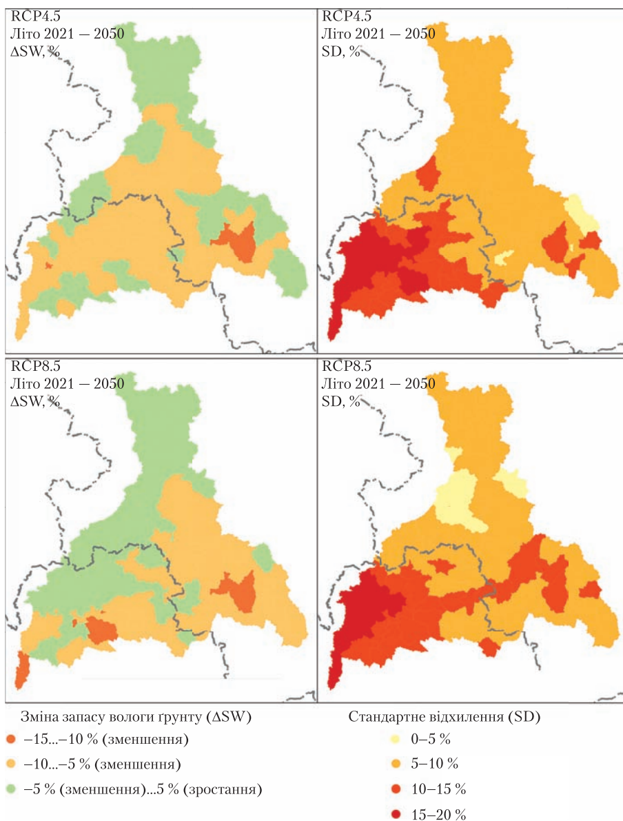
Рис. 3. Прогнозована зміна запасу вологи ґрунту басейну Десни в період 2021–2050 рр. відносно 1991–2020 рр. за сценаріями RCP4.5 та RCP8.5 за результатами моделювання SWAT: середнє (%) та стандартне відхилення (%) ансамблю регіональних кліматичних моделей
