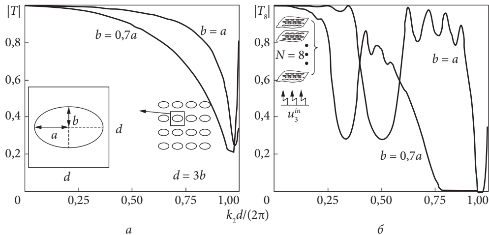
Залежності модуля коефіцієнта проходження хвиль від безрозмірного хвильового числа для: a — одноплощинного, b — восьмиплощинного тріщинного бар'єру з дво-періодичних еліптичних ( b = 0,7a ) та кругових ( b = a ) тріщин з міжгратковою відстанню ( d = 3b )
