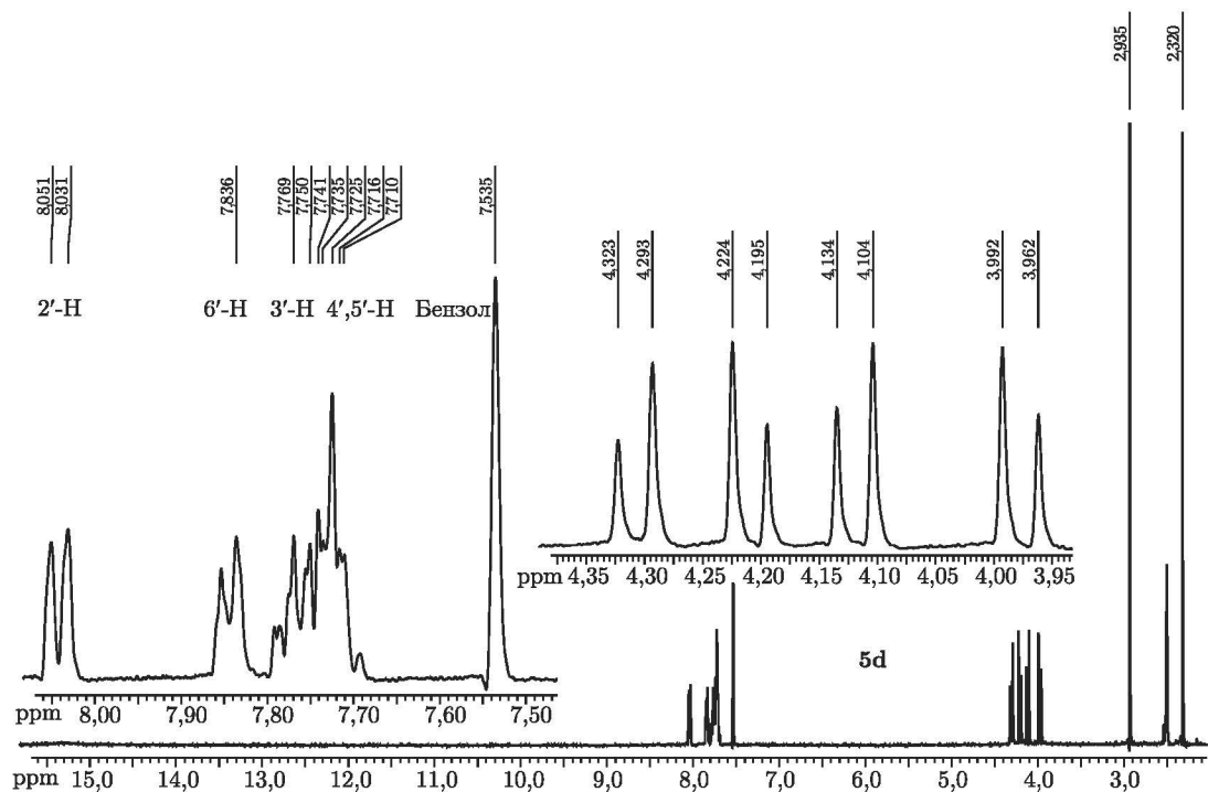
Рис. 3. Вид спектра на ядрах ^1H соединения 5d в смеси ДМСО- d_6 — C_6D_6 в соотношении 1 : 2
