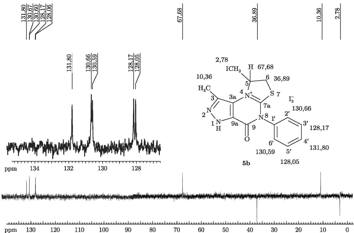
Рис. 2. Спектр АРТ соединения 5b в ДМСО- d_6 . Сигналы групп CH и CH_3 направлены вверх, а сигналы групп CH_2 — вниз
