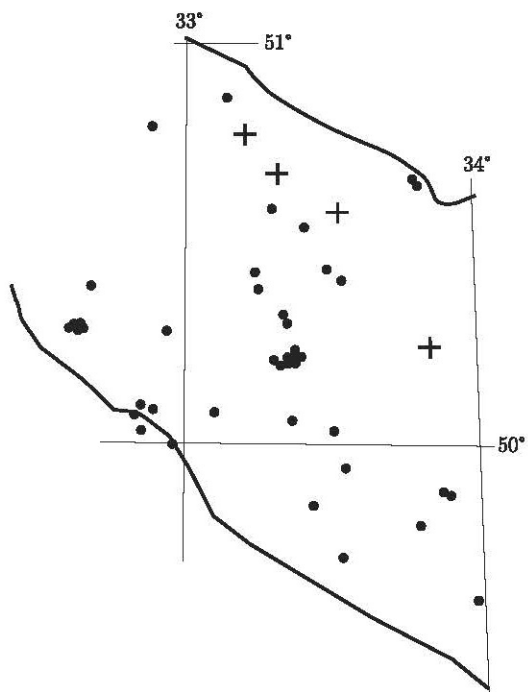
Рис. 4. Распределение в регионе пунктов с величиной ТП 50 и более мВт/м 2 (точки) и зон anomalously высоких пластовых давлений (кресты) [3]
