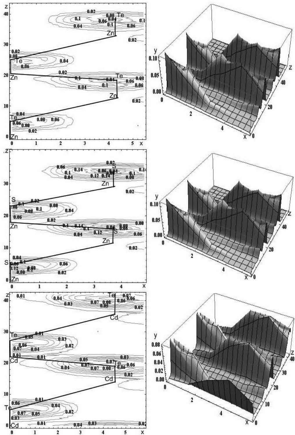
Рис. 4. Контурные карты и 3D-графики распределения плотности заряда валентных электронов в плоскости (110), перпендикулярной поверхности (111). Верхний ряд относится к ZnTe, средний — к ZnS, нижний — к CdTe. На оси y отложена плотность заряда \rho(\vec{r}) (у. е.)
