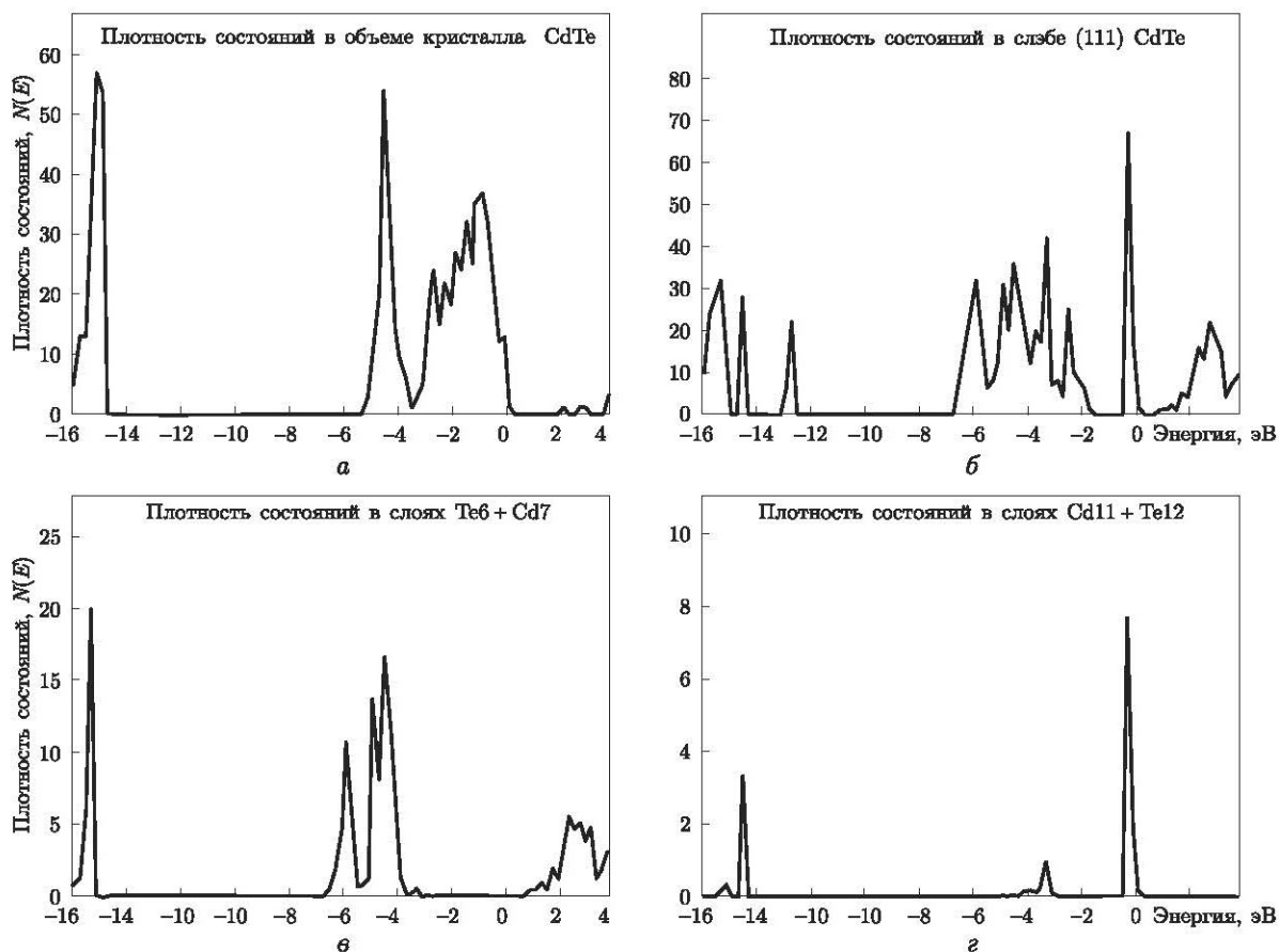
Рис. 3. CdTe: а — плотность электронных состояний в кристалле со структурой сфалерита; б — полная плотность состояний в 16-ти слойной (111) пленке; в — плотность состояний в слоях Te6 + Cd7; г — плотность состояний в поверхностных слоях Cd11 + Te12
