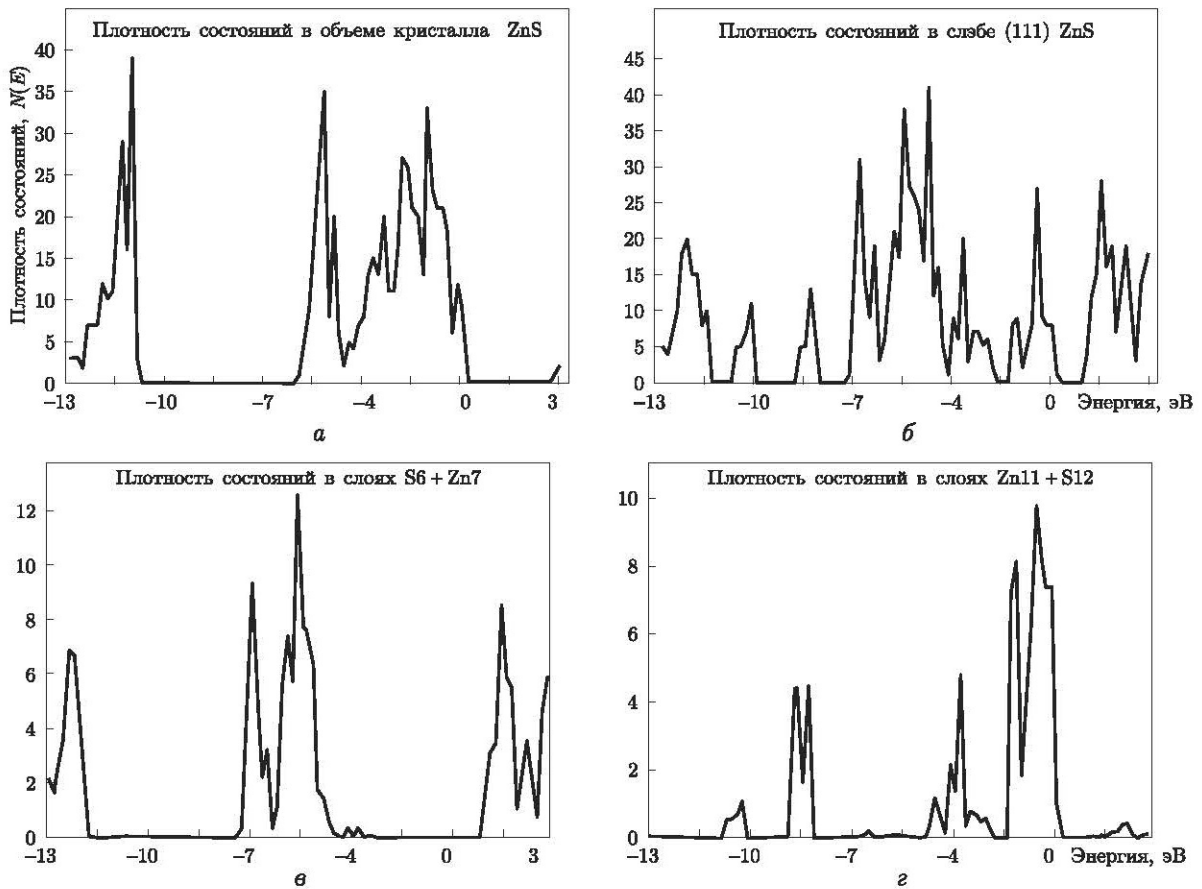
Рис. 2. ZnS: a — плотность электронных состояний в кристалле со структурой сфалерита; б — полная плотность состояний в 16-ти слойной (111) пленке; в — плотность состояний в слоях S6+Zn7; г — плотность состояний в поверхностных слоях Zn11+S12
