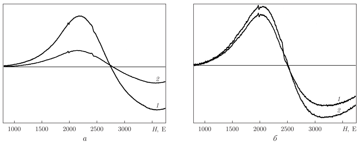
Рис. 2. Спектри ЕПР МНК (а) та \text{Fe}_3\text{O}_4 (б) при 38^\circ\text{C} . H — напруженість магнітного поля. Індукція ПМП ( B ) при активації/синтезі в реакторі: 1 — 5 мТл; 2 — 8 мТл
