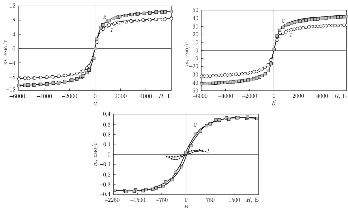
Рис. 1. Петлі гістерезису МНК (а), \text{Fe}_3\text{O}_4 (б) та ДР (в) при 38^\circ\text{C} . H — напруженість магнітного поля; m — магнітний момент. Індукція ПМП ( B ) при активації/синтезі в реакторі: 1 — 5 мТл; 2 — 8 мТл
