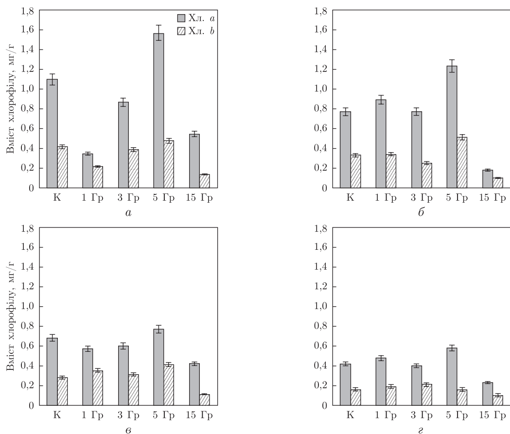
Рис. 1. Динаміка хлорофілу a та хлорофілу b (мг/г сирої маси) в онтогенезі листя Linum usitatissimum , опроміненого різними дозами рентгенівської радіації. Стадія онтогенезу листка: a — початкова (C1); б — середня (C2); в — початок в'янення (C3); г — кінцева (C4); К — контроль
