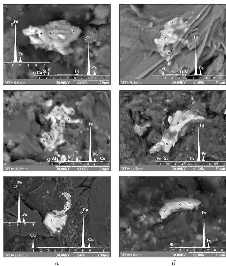
Рис. 2. Различные проявления самородного железа: а — в виде сростков с самородной медью (Fe и Cu — без заметных примесей); б — в виде частиц (с примесями Cr, Ti, V и других элементов) различной морфологии
