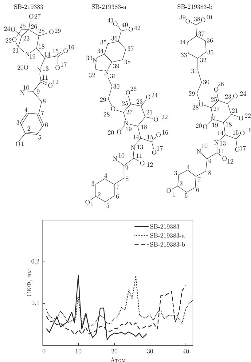
Рис. 2. Середньоквадратичні флуктуації важких атомів інгібіторів MtTyrRS у ході динаміки. Пікові значення флуктуацій не перевищують 2 Å
