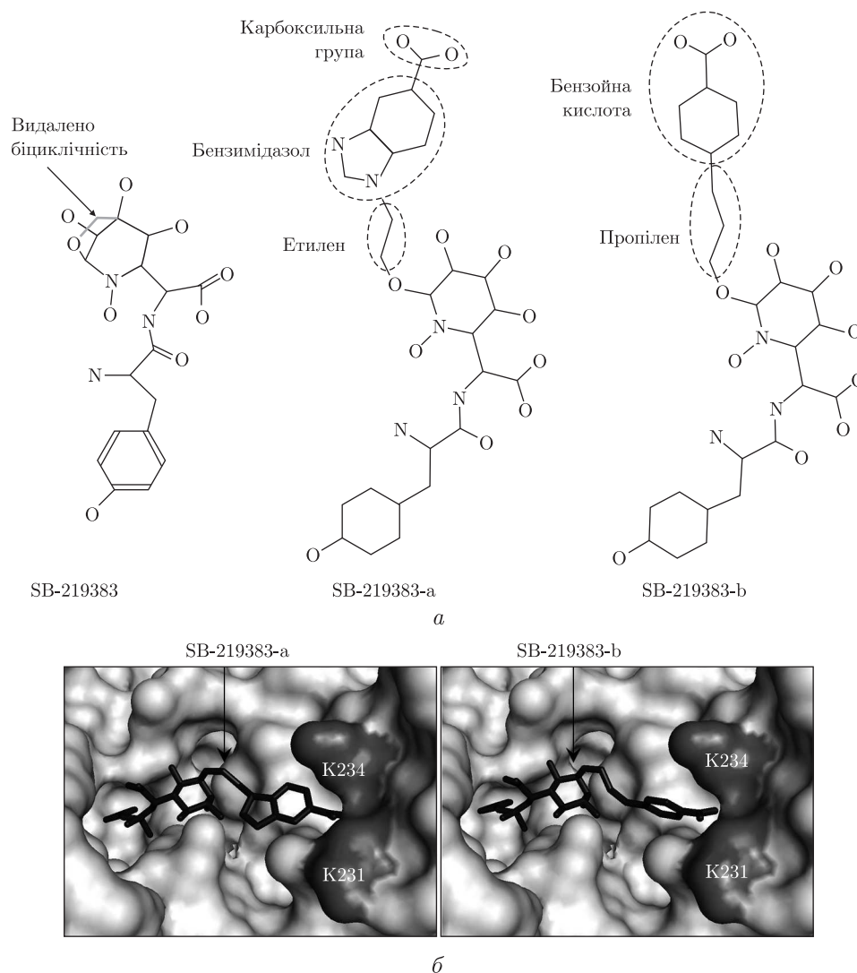
Рис. 1. Інгібітор SB-219383 та побудовані його аналоги: для першого змодельованого інгібітора видалено біциклічність і приєднано до атома оксигену етиленовий фрагмент, бензimidазол та карбоксильну групу (SB-219383-a), для другого інгібітора до атома оксигену приєднано пропіленовий фрагмент і бензойну кислоту (SB-219383-b) (a). Поверхня кишені активного центру Mt TyrRS та побудовані інгібітори: інгібітори займають всю кишеню активного центру Mt TyrRS та взаємодіють з каталітичною петлею KFGKS; карбоксильні групи інгібіторів мають електростатичні взаємодії з каталітичними залишками лізину Lys231 та Lys234 (б)
