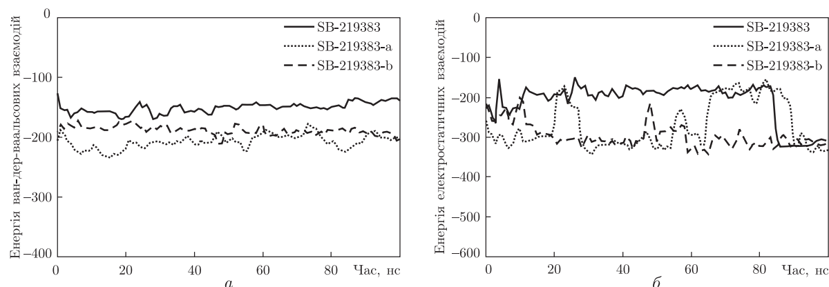
Рис. 3. Енергія взаємодії інгібіторів з ферментом в активному центрі: значення енергії ван-дер-ваальсових взаємодій інгібіторів SB-219383-a та SB-219383-b є нижчими, ніж у інгібітора SB-219383, що зумовлено більшою площею взаємодіючої поверхні (а). Енергія електростатичних взаємодій інгібіторів з ферментом (б). Значення енергій для нових інгібіторів загалом є нижчим порівняно з SB-219383. На 85-й нс динаміки SB-219383 формує водневі зв'язки із зарядженим залишком Asp40, що істотно відбивається на значеннях енергії. Таким чином, на проміжку динаміки 85–100 нс величини енергії для всіх трьох інгібіторів знаходяться в межах \approx -250 \div -400 кДж/моль
