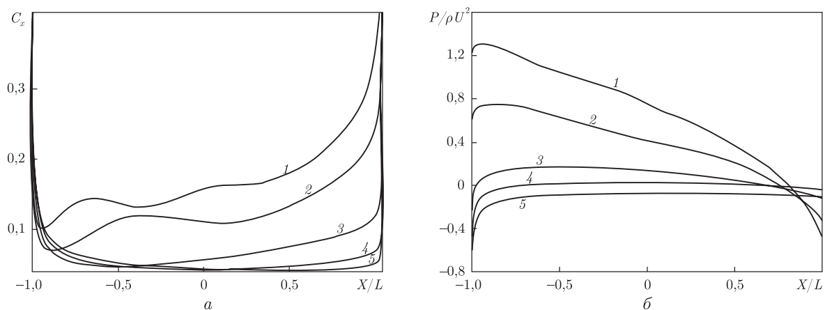
Рис. 3. Распределения коэффициента сопротивления трения (а) и давления (б) вдоль верхней стороны пластины ( L = 10 см, h = 0,5 см) для различных значений числа Фруда: Re = 500 , Fr = 0,05; 0,125; 0,5; 5000 (кривые 1–5)
