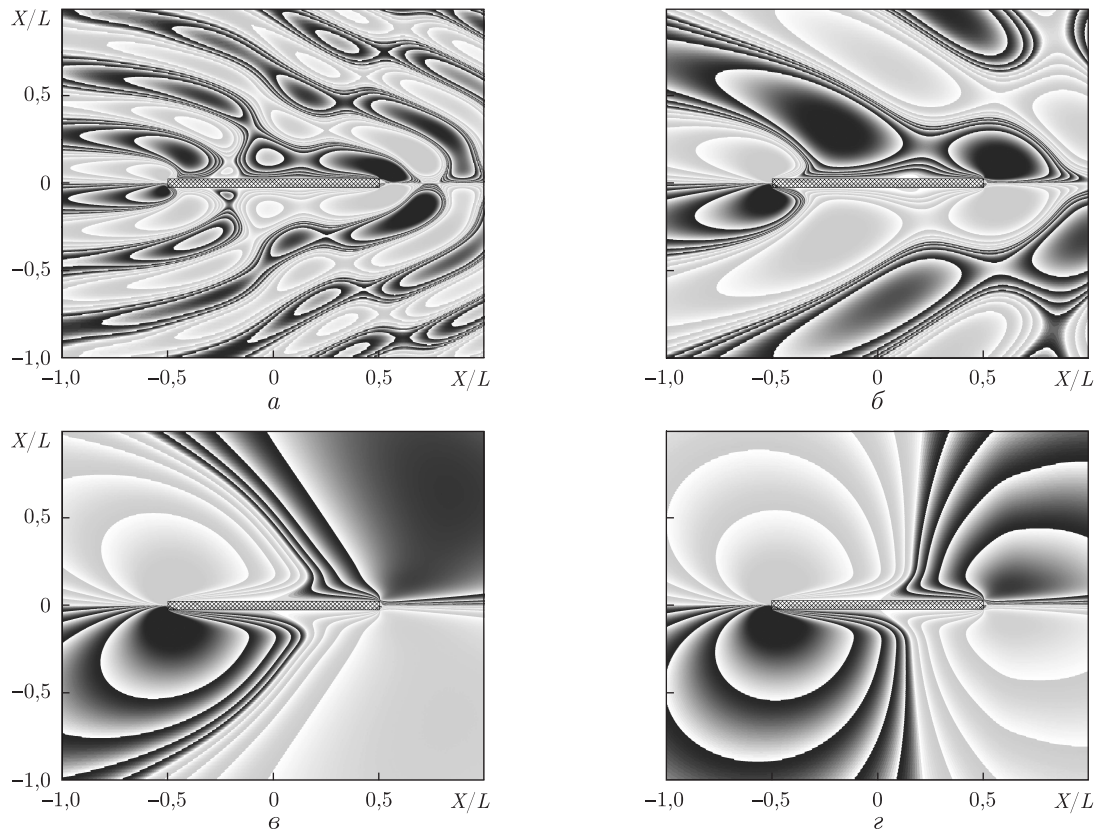
Рис. 1. Поля вертикальной компоненты скорости жидкости около горизонтальной пластины ( L = 10 см, h = 0,5 см), обтекаемой потоком стратифицированной жидкости для различных значений числа Фруда при Re = 500 : а-г — Fr = 0,05 ; 0,125 ; 0,5 ; 5000
