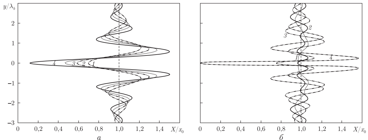
Рис. 2. Деформации плотностных маркеров в различных сечениях впереди (а) и в следе (б) за обтекаемой пластиной ( L = 10 см, h = 0,5 см): Re = 500 , Fr = 0,05 , |x_0/L| = 1,5; 1,0; 0,75; 0,53 (кривые 1–4)
