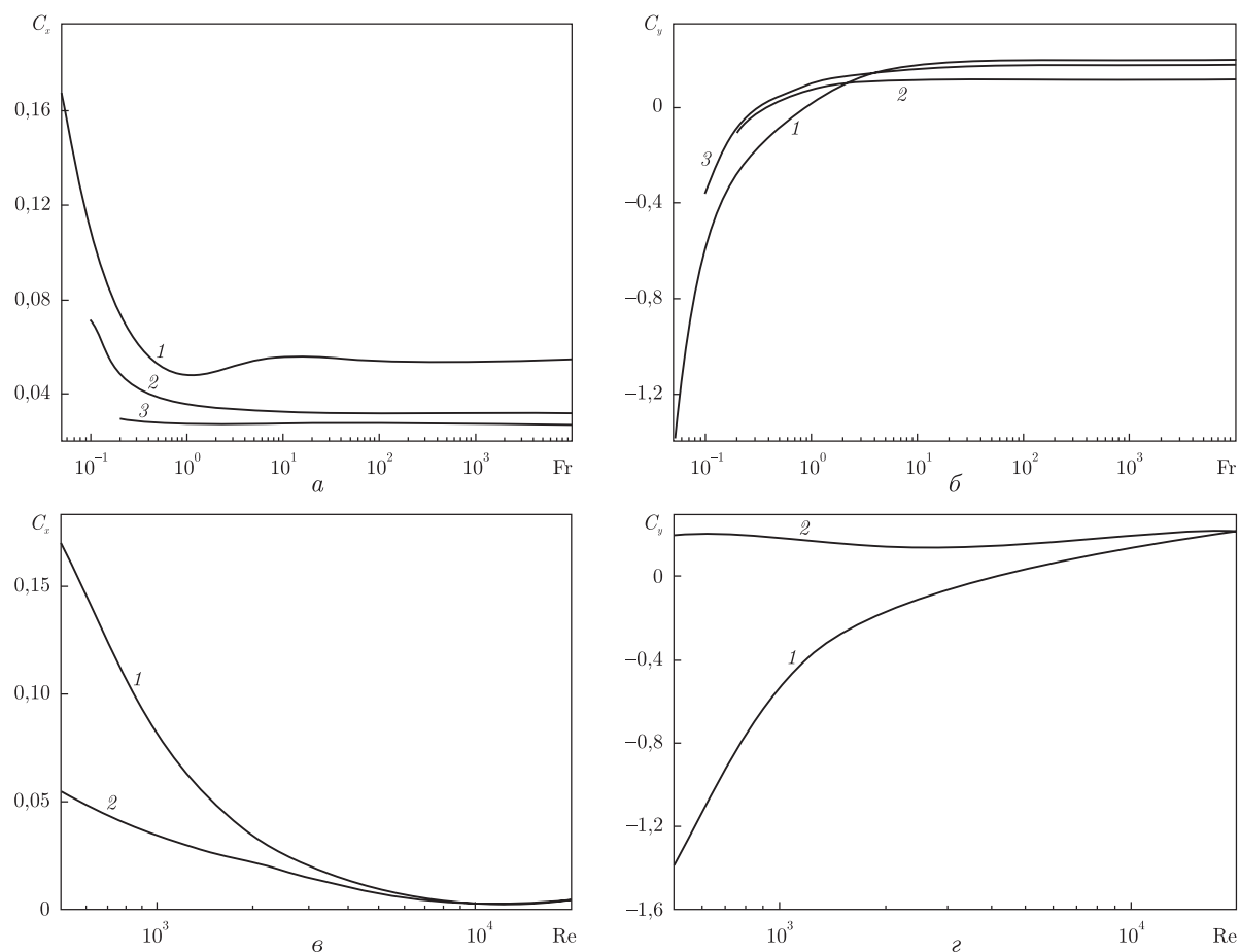
Рис. 4. Интегральные значения коэффициентов сопротивления трения (а, б) и подъемной силы (б, з), действующих на верхнюю сторону пластины, как функции числа Фруда (а, б) при Re = 500; 1000; 2000 (кривые 1–3) и числа Рейнольдса (в, з) при Fr = 0,05; 5000 (кривые 1, 2)
