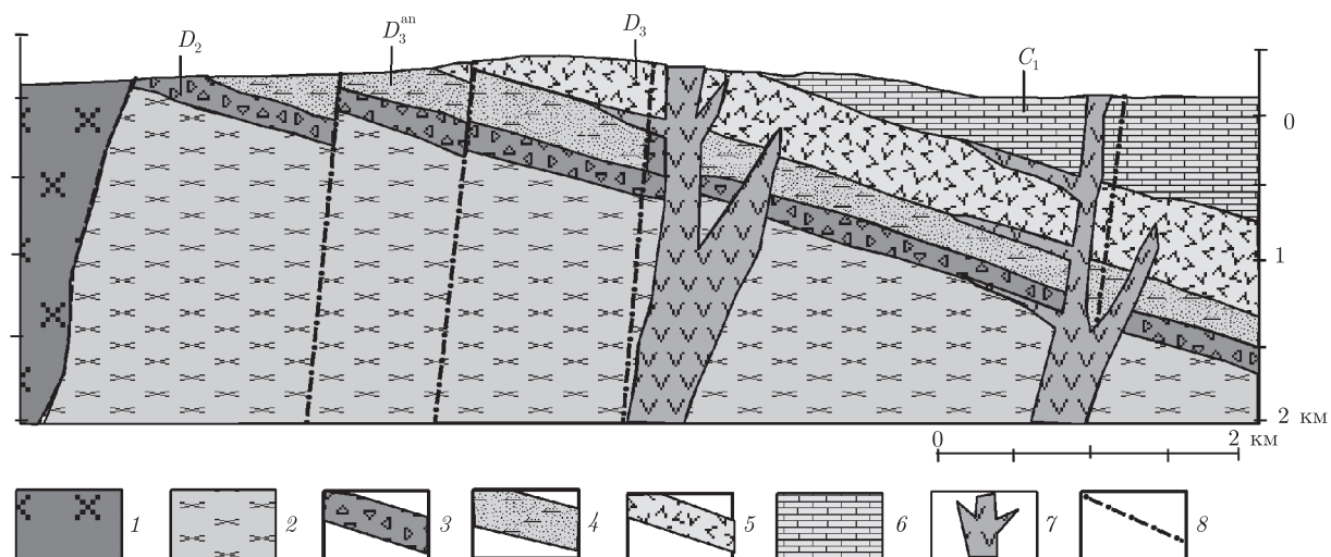
Рис. 1. Схематический геологический разрез района внедрения Новоигнатьевской дайки андезитовых порфиритов:
