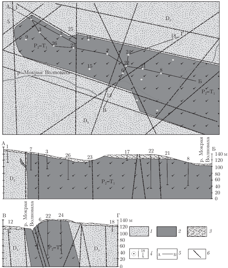
Рис. 2. Схематический план и геологические разрезы (по линии А–Б и В–Г) Новоигнатьевской дайки андезитовых порфириров:
