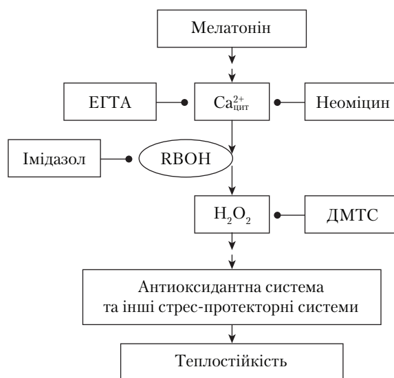
Рис. 4. Гіпотетична схема \text{Ca}^{2+} - і АФК-залежного впливу мелатоніну на теплостійкість проростків пшениці. RBOH — каталітична субодиниця НАДФН-оксидази. Пояснення в тексті
