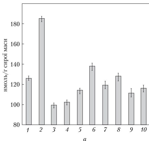
Рис. 3. Вміст пероксиду водню в коренях (а) і вживаність проростків пшениці (б) після ушкоджувального прогріву (45 °С, 10 хв) за їх оброблення мелатоніном, ДМТС, імідазолом та антагоністами кальцію. 1 – контроль; 2 – мелатонін (1 мкМ); 3 – ДМТС (150 мкМ); 4 – мелатонін (1 мкМ) + ДМТС (150 мкМ); 5 – імідазол (10 мкМ); 6 – мелатонін (1 мкМ) + імідазол (10 мкМ); 7 – ЕГТА (500 мкМ); 8 – мелатонін (1 мкМ) + ЕГТА (500 мкМ); 9 – неоміцин (200 мкМ); 10 – мелатонін (1 мкМ) + неоміцин (200 мкМ)
