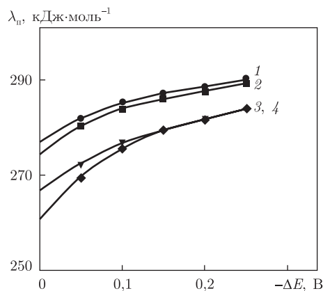
Рис. 3. Зависимость полной энергии реорганизации системы от перенапряжения в гидроксипалладиоиминодиацетатном электролите палладирования при температуре, °С: 22 (1), 30 (2), 40 (3), 50 (4)
