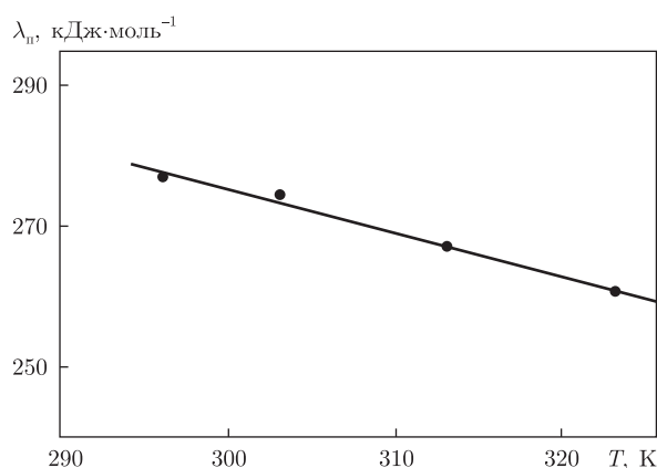
Рис. 4. Зависимость полной энергии реорганизации системы в гидроксипалладиоиминодиацетатном электролите палладирования от температуры
