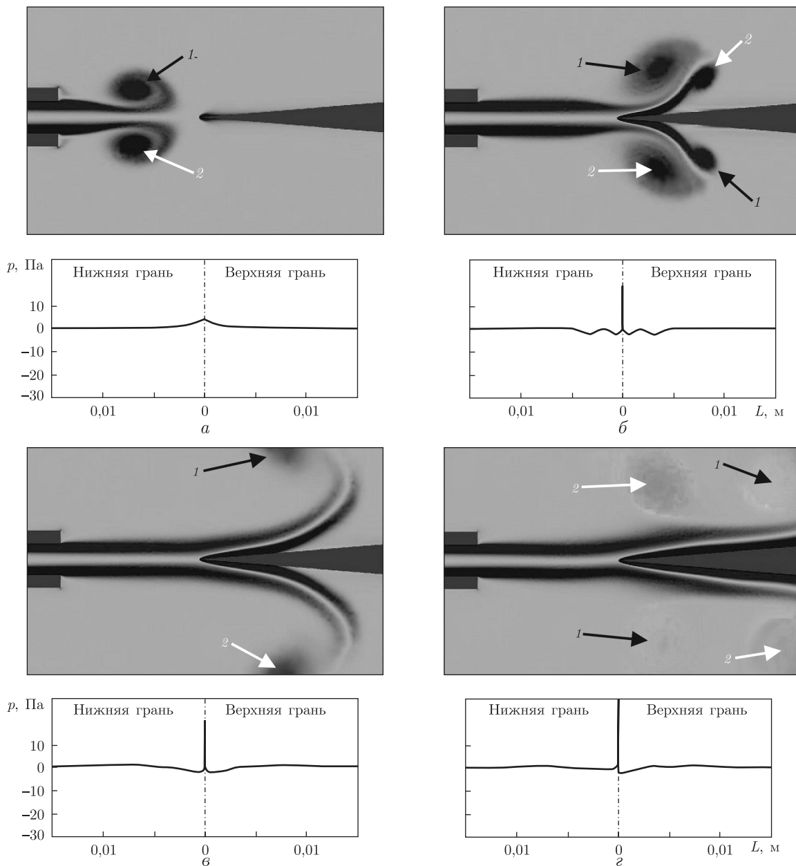
Рис. 3. Поле завихренности и распределение давления на поверхностях клина в течение переходного процесса: 1 — области положительной завихренности, т.е. жидкость закручивается против часовой стрелки; 2 — области отрицательной завихренности, т.е. жидкость закручивается по часовой стрелке
