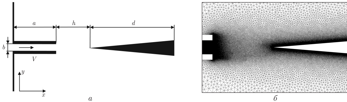
Рис. 1. Геометрия задачи: а — расчетная область; б — триангулярная сетка, на которой проводилась пространственная дискретизация
