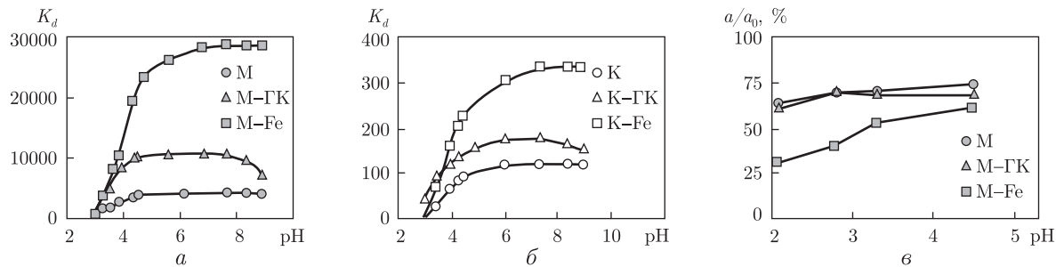
Рис. 1. Влияние pH водного раствора на сорбционно-десорбционные процессы цезия из монтмориллонитовых (а, в) и каолиновых (б) образцов
