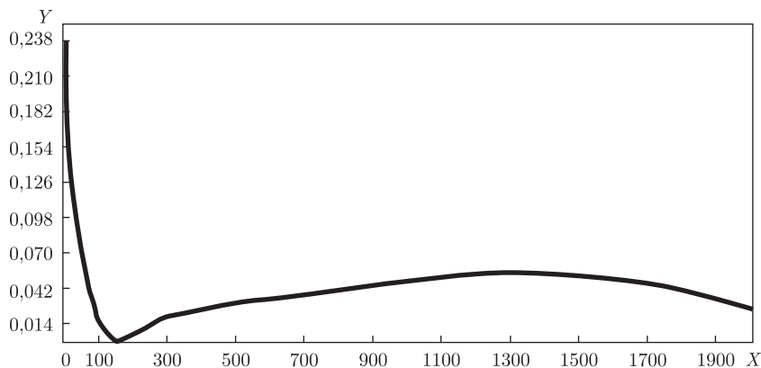
Рис. 1. Осереднена залежність змін модулів швидкості течій з глибиною. Вісь Y — швидкість, м/с; X — глибина, м
