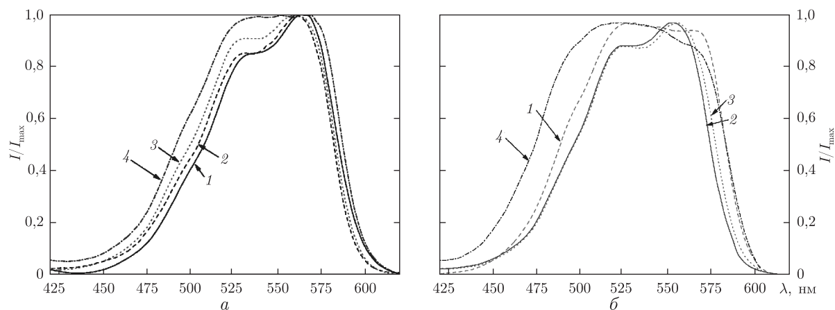
Рис. 2. Нормированные спектры возбуждения флуоресценции пленок ГКБЭ + ПК 5 (1), ПК 4 (2), ПК 1 (3), ПК 6 (4); массовая концентрация ПК 1% (а) и 10% (б); \lambda_{\text{рег.}} = 700 нм
