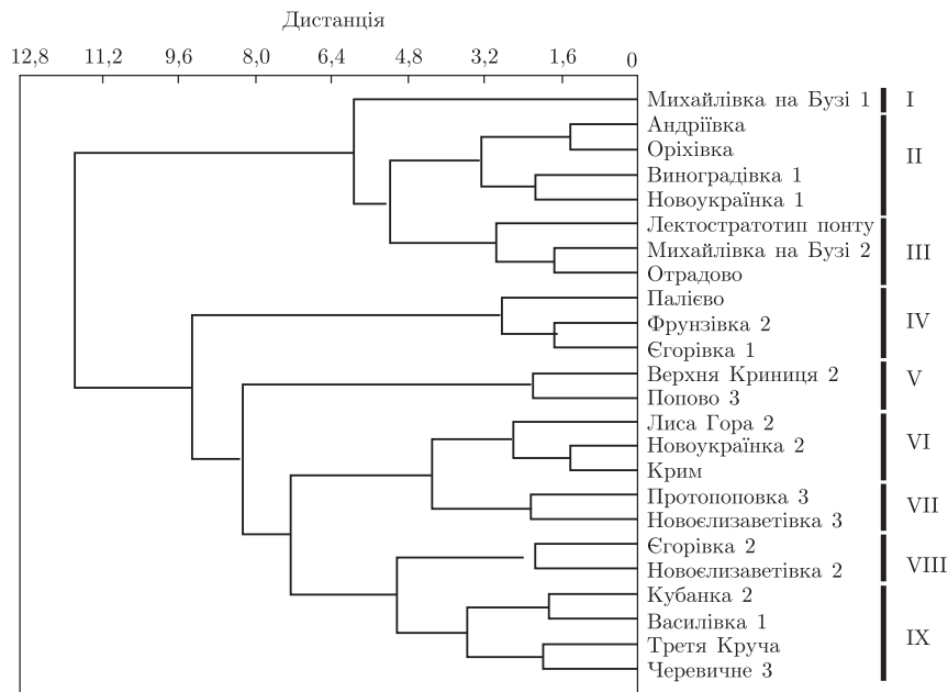
Рис. 1. Дендрограма подібності угруповань іхтіофауни пізнього міоцену півдня України (ієрархічний кластерний аналіз за методом Варда)
