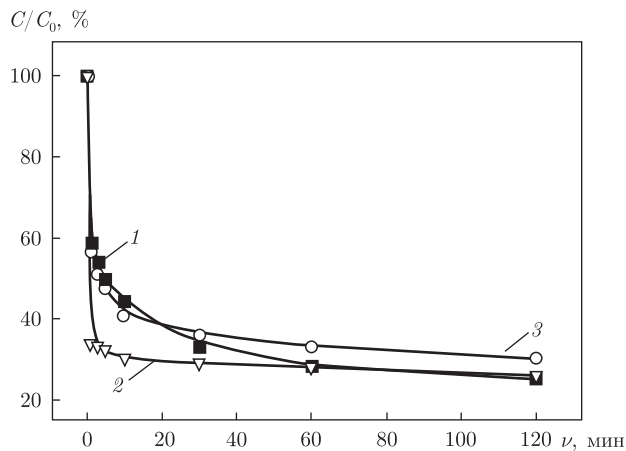
Рис. 1. Кинетические кривые гибели радикала ДФПГ в реакции с экстрактами Vitex negundo var. cannabifolia (1), Vitex agnus-castus (2), Vitex negundo (3). Разбавление исходных экстрактов 1 : 50 [ \tau — время, ч; C/C_0 — отношение концентрации радикала в растворе к исходной концентрации, %]
