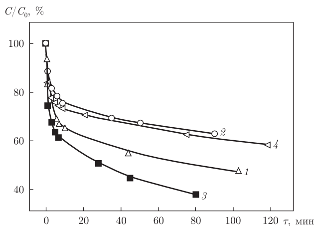
Рис. 2. Кинетические кривые гибели радикала ДФПГ в реакции с экстрактами Magnolia sieboldii (1), Magnolia kobus (2), Magnolia x soulangeana (3), Magnolia stellata (4). Разбавление исходных экстрактов 1 : 40 [ \tau — время, ч; C/C_0 — отношение концентрации радикала в растворе к исходной концентрации, %]
