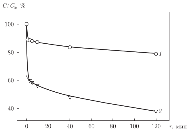
Рис. 4. Кинетические кривые гибели радикалаДФПГ в реакции с экстрактами из листьев растений Stevia rebaudiana , выращенных в открытом грунте (1) и в системе in vitro (2). Разбавление исходных экстрактов 1 : 50 [ \tau — время, ч; C/C_0 — отношение концентрации радикала в растворе к исходной концентрации, %]
