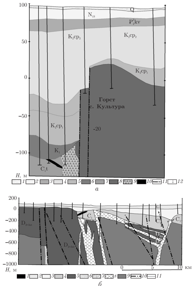
Рис. 2. Геологический разрез:
