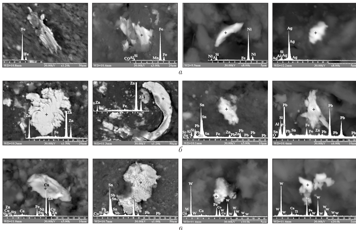
Рис. 4. ДСМЧ в визейских ЧС центральной части Днепровско-Донецкой впадины: а — частицы самородного железа, никеля, серебра (Свиридовская скв. 5, гл. 5830–5842 м); б — частицы цинка, олова и их сросток (Бельская скв. 470, гл. 4666–4674 м); в — частицы природных сплавов меди и цинка с примесью железа и никеля (латунь-бронза); олова и меди (бронза); вольфрама — железа — кобальта; вольфрама — железа — титана (Божковская скв. 1, гл. 5056–5063 м)
