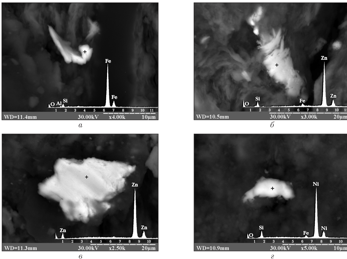
Рис. 1. ДСМЧ в менилитовых сланцах (с. Синевидное): а — самородное железо; б — самородный цинк (с примесью железа); в — самородный цинк; г — самородный никель (с примесью железа)
