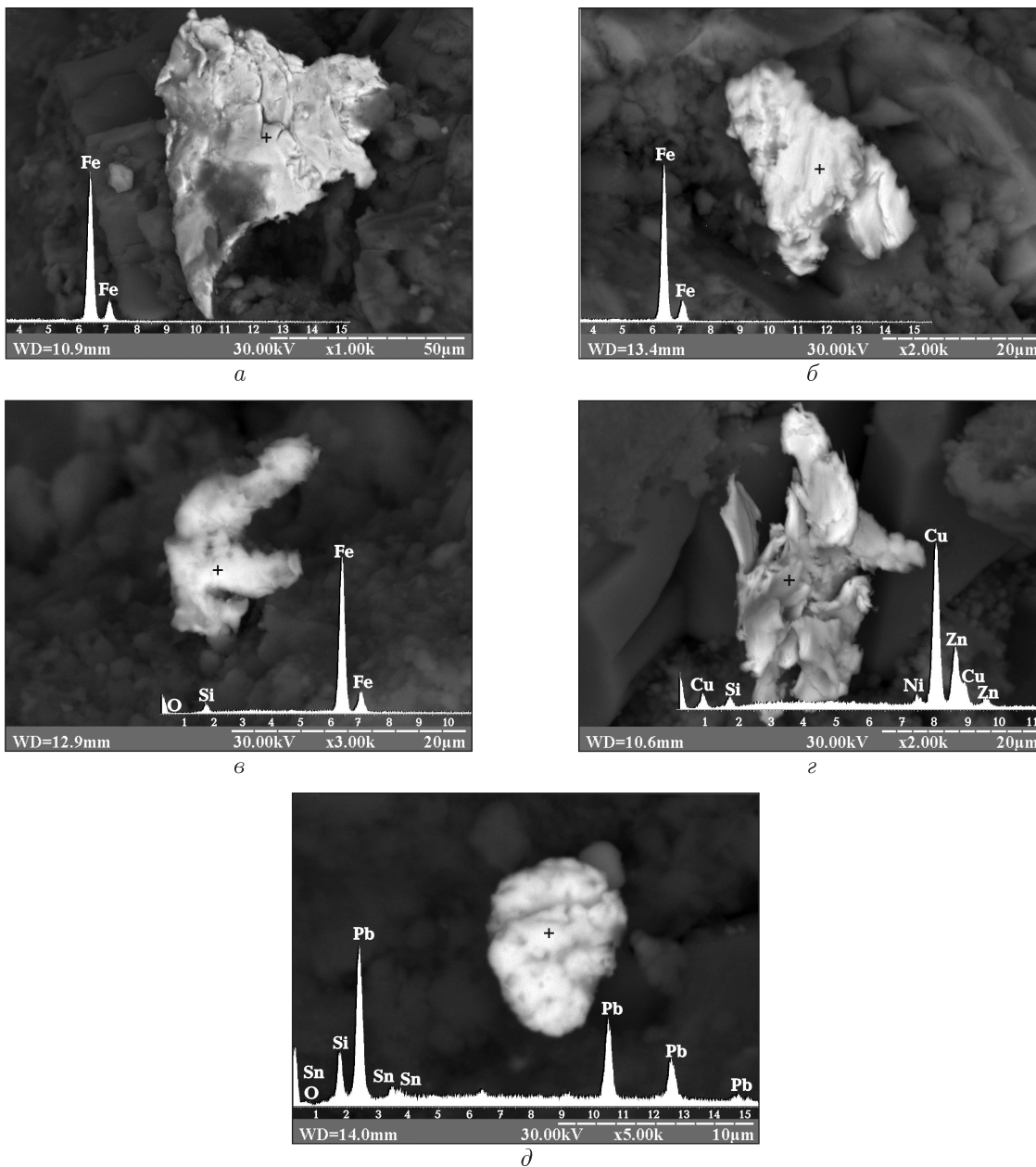
Рис. 3. ДСМЧ в майкопских ЧС Прикерченского шельфа (месторождение Субботина): а ... в — самородное железо ( а — скв. 1, гл. 2500–2506 м; б — скв. 1, гл. 2498–2503 м; в — скв. 403, гл. 2439–2444 м); г — цинкистая медь (природная латунь) с примесью никеля (скв. 1, гл. 2490–2495 м); д — свинец с примесью олова (скв. 403, гл. 2591–2596 м)
