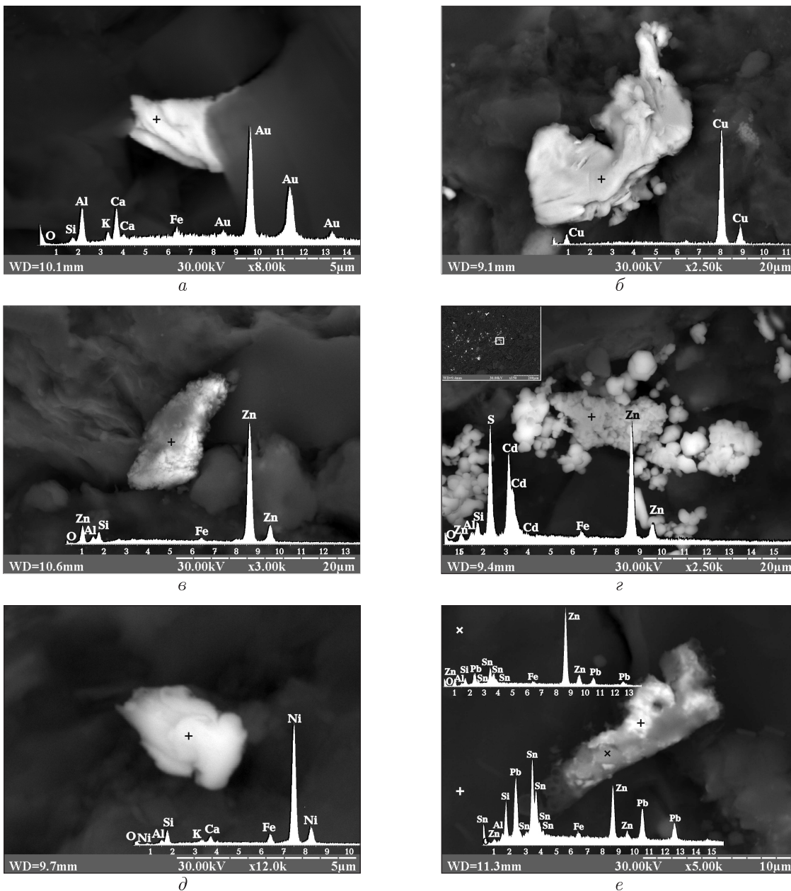
Рис. 2. ДСМЧ в силурийских ЧС Львовского прогиба: а — золото (Великомостовская скв. 30, гл. 3867–3873 м); б — медь (Великомостовская скв. 30, гл. 3867–3873 м); в — цинк (с примесью железа) (Великомостовская скв. 30, гл. 4017–4025 м); г — ассоциация самородного цинка с кадмийсодержащим сфалеритом (пшибрамитом) (Великомостовская скв. 30, гл. 4017–4025 м); д — никель с примесями железа (Глинянская скв. 1, гл. 2334–2339 м); е — агрегат частиц природного сплава цинка, свинца и олова с различными соотношениями указанных металлов и примесью железа (Добровторская скв. 1, гл. 3216–3221 м)
