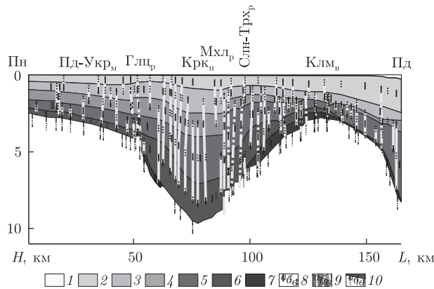
Рис. 2. Сейсмоструктурний розріз уздовж профілю: Пд-Укр м — Південно-Українська монокліналь, Крк п — Каркінітський прогін, Клм в — Каламітський вал. Розломи: Глц — Голіцинський, Мхл — Михайлівський, Слн-Трх — Сулінсько-Тарханкутський. Умовні позначення: 1 — вода; осадові шари: 2 — середній міоцен — голоцен ( N_1^2-Q ), 3 — майкопська світа ( P_3-N_1^1 ), 4 — палеоцен — еоцен ( P_{1-2} ), 5 — верхня крейда ( K_2 ), 6 — нижня крейда ( K_1 ), 7 — догер-мальм ( J_2-3 ); 8 — засічки, що відзначають точки перегинів графіків V_{oc} : а — локальні максимуми, б — локальні мінімуми, в — стрибки швидкості; 9 — виділені розломи: а — в осадовому чохлі, б — що виходять у фундамент, в — зафіксовані сейсмікою; 10 — положення розломів за літературними даними: а — за [2], б — за [5], в — за [6]
