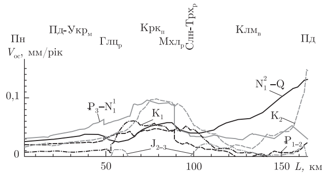
Рис. 3. Графіки швидкостей осадконагромадження вздовж профілю № 568408 у мезокайнозой
