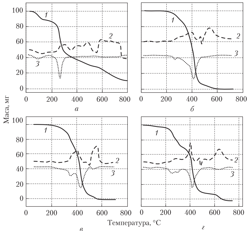
Рис. 3. Криві диференціального термогравіметричного аналізу Кс (а), ІПУ (б), ІПУ/РО40 (в) та ІПУ/РО40/Кс20 (г): 1 – ТГ; 2 – ДТА; 3 – ДТГ
