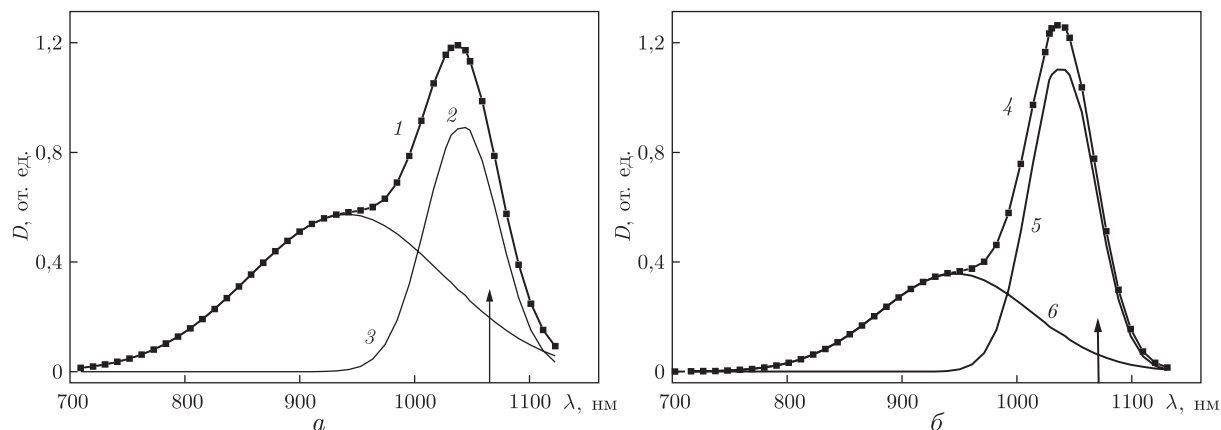
Рис. 4. Графическое разделение полос поглощения ПК: а – в ПУ-1, б – в ПУ-2 (1, 4 – исходные кривые, 2, 5 – мономерная форма, 3, 6 – димерная форма)
