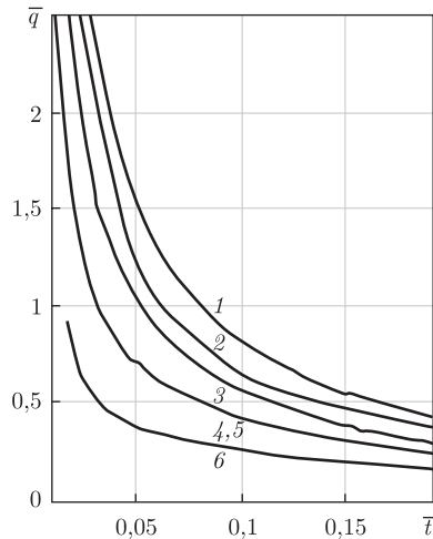
Рис. 3. Относительный фильтрационный расход при увлажнении колонки грунта: 1, 3 – грунт I; 2, 4 – грунт II; 5, 6 – грунт III; 1, 3, 4, 6 – по (15), (17); 1 – при a_w = 0 ; 3, 4, 6 – при a_w > 0 ; 1, 2, 5 – по (17), (18)
