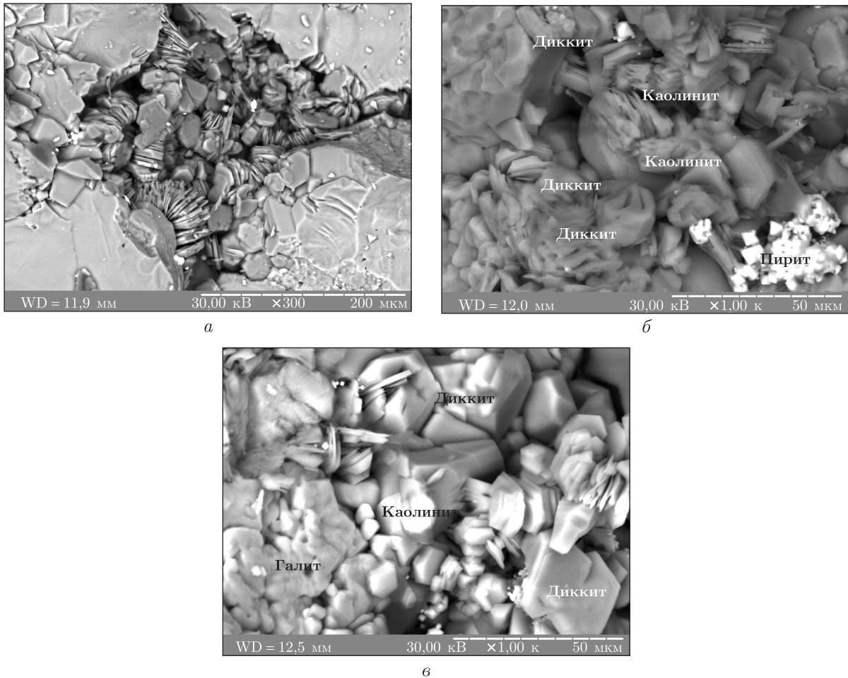
Рис. 4. Особенности морфологии и минерального состава вторичных пор-каверн, заполненных микропористым диккит-каолиновым кристаллическим агрегатом в парагенезе с пиритом и галитом (ДДВ, скв. С-17, инт. 6527,7–6531,6 м)
