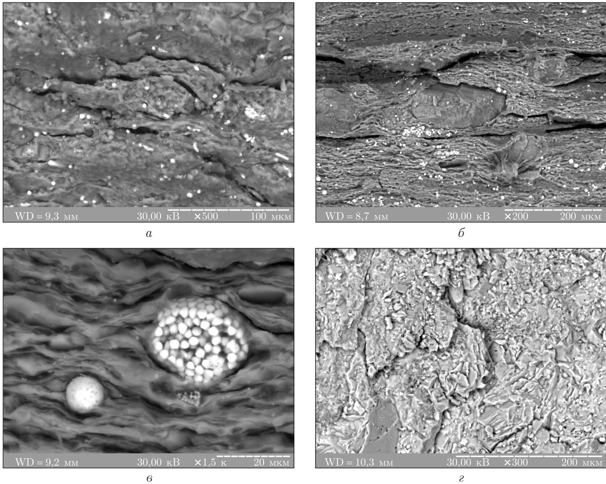
Рис. 2. Открытая прерывистая микротрещиноватость в милонитизированном черном сланце ( а, б, в ) и в перекристаллизованном известняке ( г ). ДДВ, скв С-17: а — инт. 5974,5–5980,58 м; б, в — инт. 6524–6527,7 м; г — инт. 6206–6210 м
