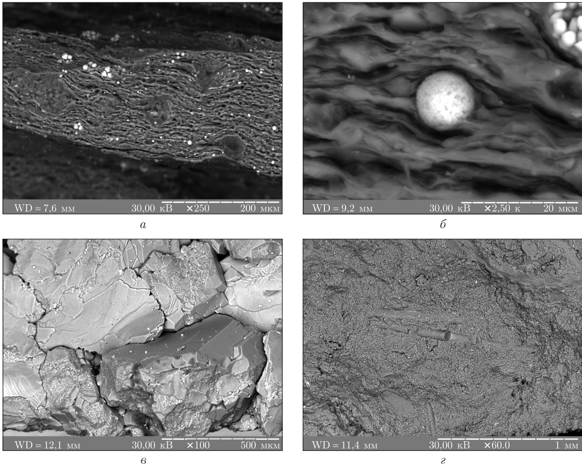
Рис. 1. Милонитизация пород глубокозалегающего верхнетурнейского комплекса (электронный микроскоп РЭМ-106 с рентгеноспектральным зондом): a, б — черный сланец (гидрокарбопелит); в — кварцитопесчаник (микростилолитизация межзерновых контактов); г — известняк (ДДВ, скв. С-17, инт. 6524–6531,6 м)
