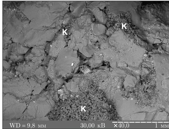
Рис. 3. Система вторичной пустотности в кварцитопесчанике (зерна кварца с признаками интенсивного сжатия): открытые поры (черное), каверны, заполненные микропористыми диккит-каолинитовыми кристаллическими агрегатами (К)
