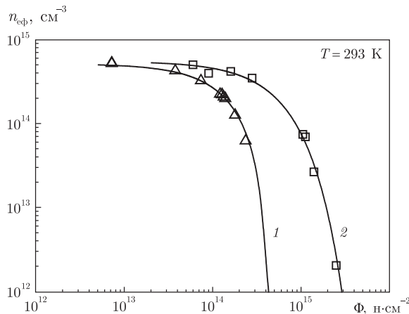
Рис. 1. Залежність ефективної концентрації носіїв ( n_{\text{еф}} ) від флюенса швидких нейтронів реактора ( \Phi ) при кімнатній температурі у зразках Cz–Si: 1 – n -Si без Ge; 2 – n -Si (Ge); \Delta – експериментальні дані; суцільні криві – результати розрахунку
