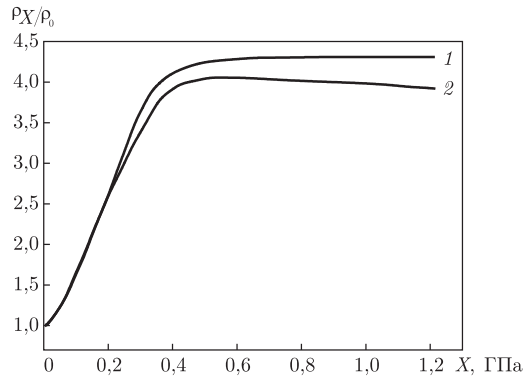
Рис. 2. Залежності тензоопору \rho_X/\rho_0 від величини механічного навантаження X , виміряні при T = 77 К, для кристалів: 1 – n -Si(P) ( \rho_{300\text{K}} \approx 55,8 Ом·см); 2 – n -Si(P + Ge) ( \rho_{300\text{K}} \approx 56,3 Ом·см)
