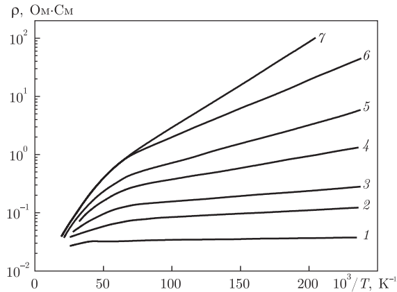
Рис. 3. Залежності питомого опору кристалів n\text{-Si(P)} ( N_P \approx 3,98 \cdot 10^{18} \text{ см}^{-3} ) від температури в інтервалі 4,2–78 К при різних значеннях \bar{X} // \bar{J} // [111] . X , ГПа: 1 – 0; 2 – 1,6; 3 – 2,0; 4 – 2,4; 5 – 2,6; 6 – 2,8; 7 – 3,0
