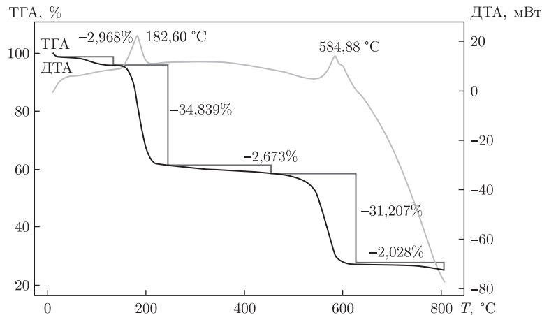
Рис. 4. Термогравіграма комплексу \text{Eu}(\text{HL})_3(\text{NO}_3)_3
