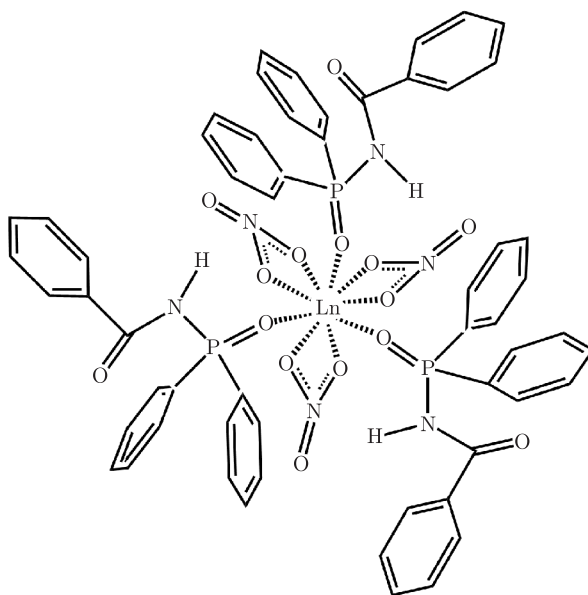
Рис. 2. Структурна формула триніtrato-трис-дифенілфосфорилбензамід лантаноїдів (III)
